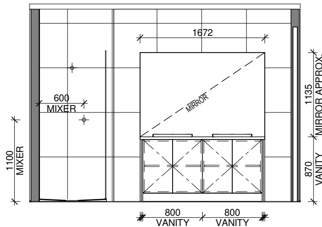
ELEVATION - E1B
