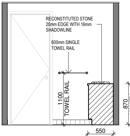
ELEVATION - E3B
