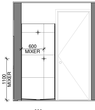
ELEVATION - E4B
