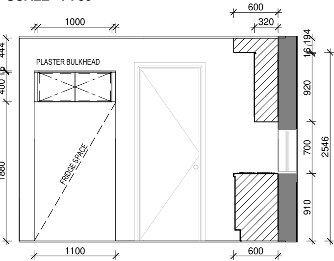
ELEVATION - KA
