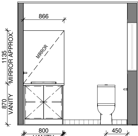
ELEVATION - E3C
