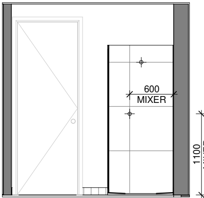
ELEVATION - E2C
