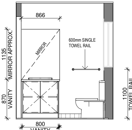
ELEVATION - E4D
