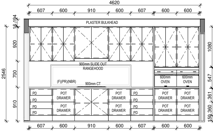
ELEVATION - KB
