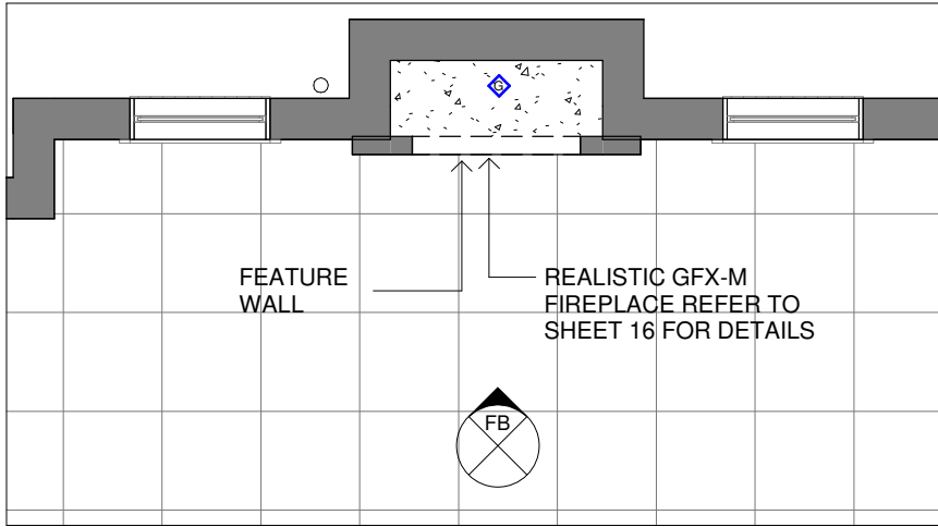
LIVING PLAN SCALE 1 : 50
