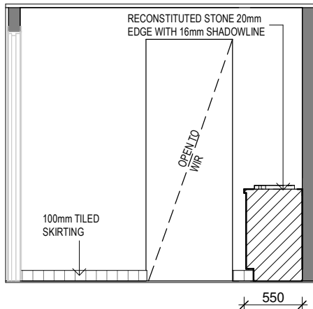
ELEVATION - E4C
