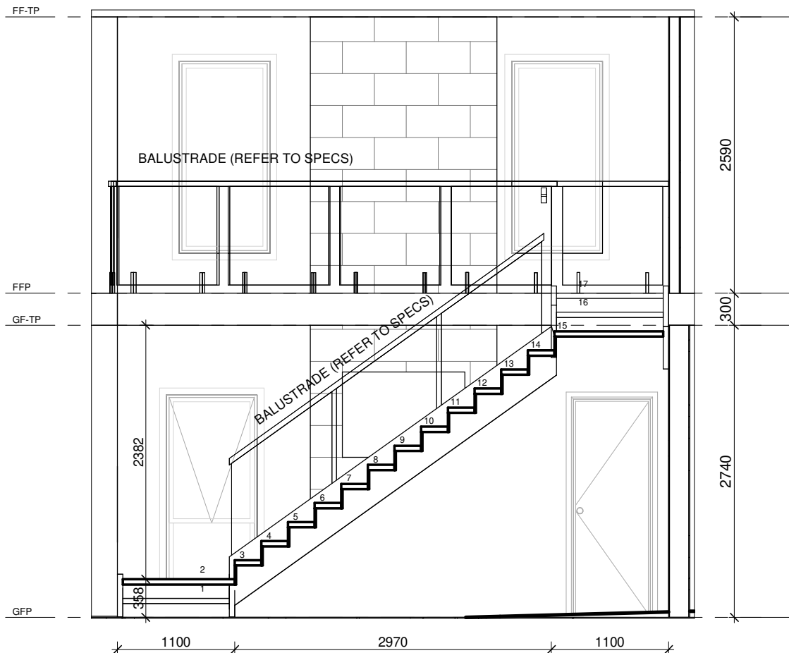
STAIR SECTION SCALE 1 : 50
