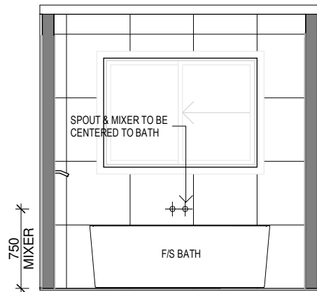
ELEVATION - E1D
