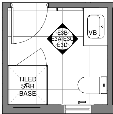
ENS 3 PLAN SCALE 1 : 50
