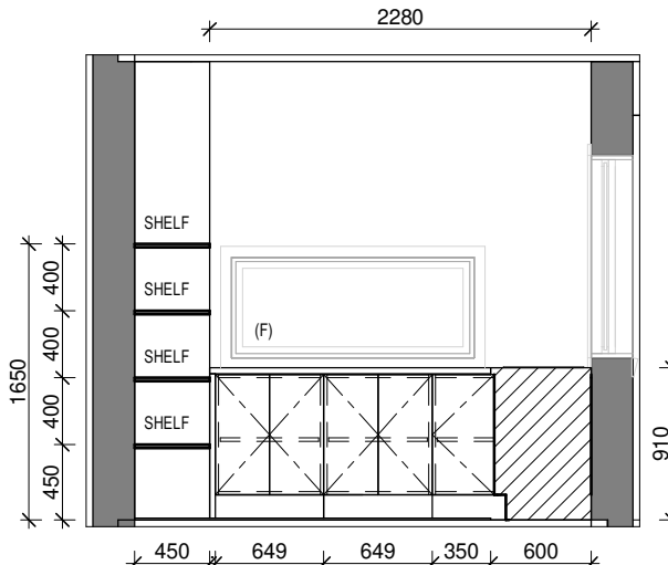
ELEVATION - KAA
