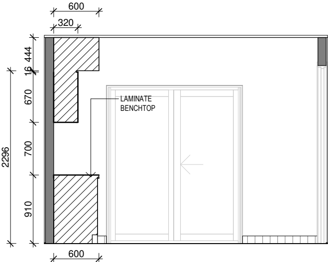
ELEVATION - LD
