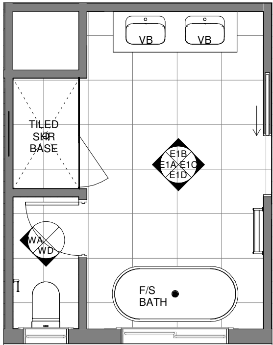
ENS 1 PLAN SCALE 1 : 50
