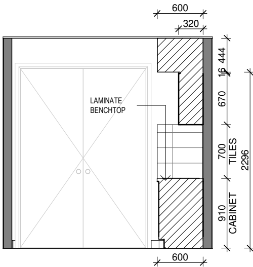
ELEVATION - LB
