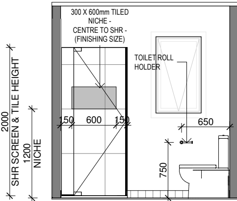
ELEVATION - E2D
