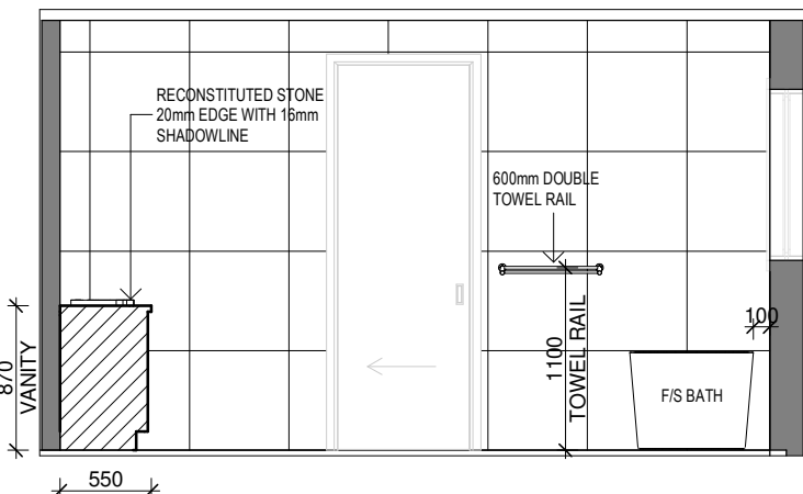
ELEVATION - E1C
