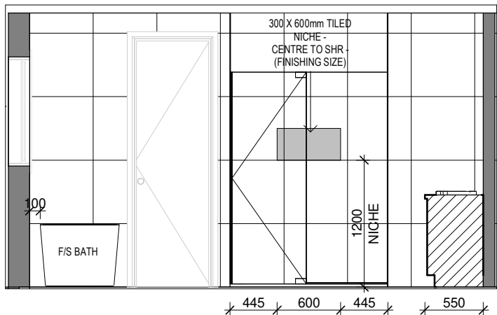
ELEVATION - E1A ENS 1 ELEVATIONS
