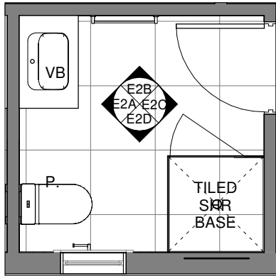
ENS 2 PLAN SCALE 1 : 50
