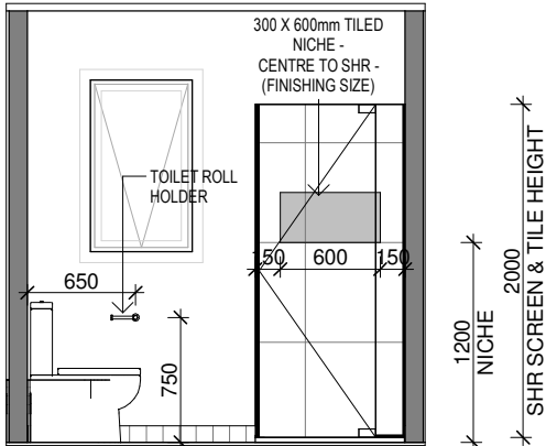
ELEVATION - E3D
