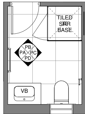
PDR PLAN SCALE 1 : 50
