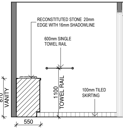
ELEVATION - E2B
