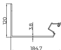
7 Louvres
