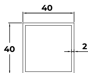
3- 40X40 PROFILE
