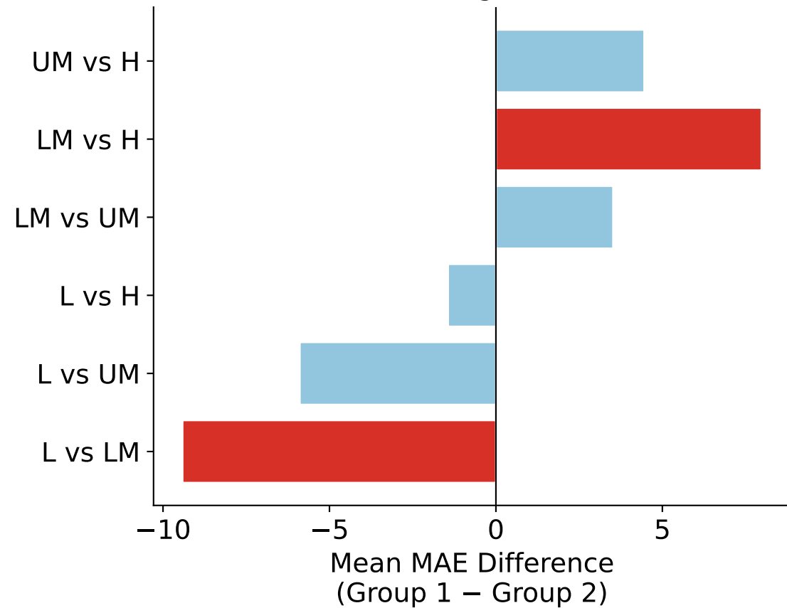
SVR
