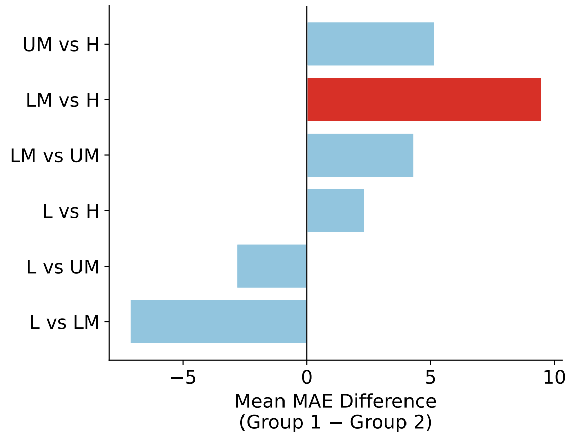
SVR
