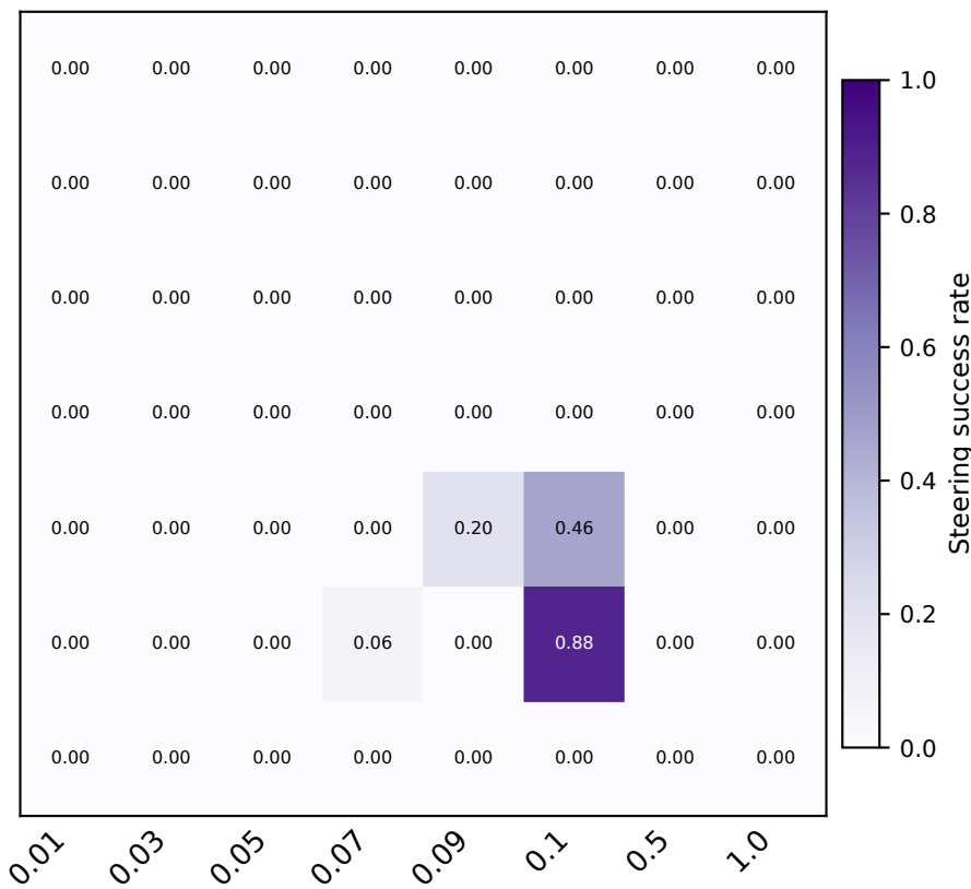
Qwen 1.5-32B
