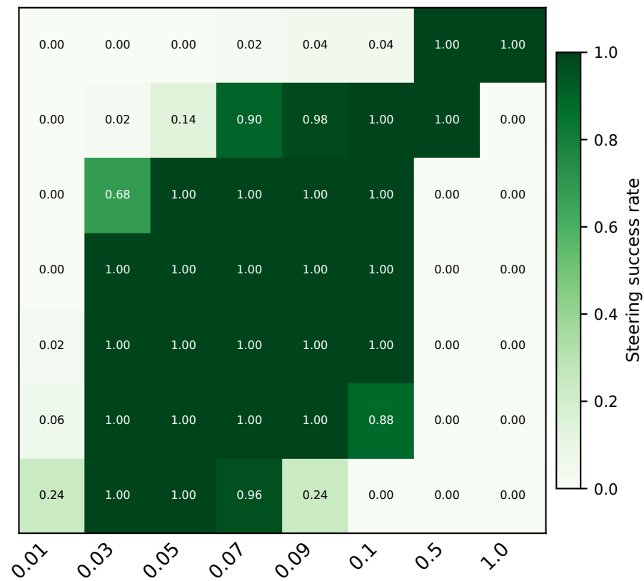
OLMo 2-13B
