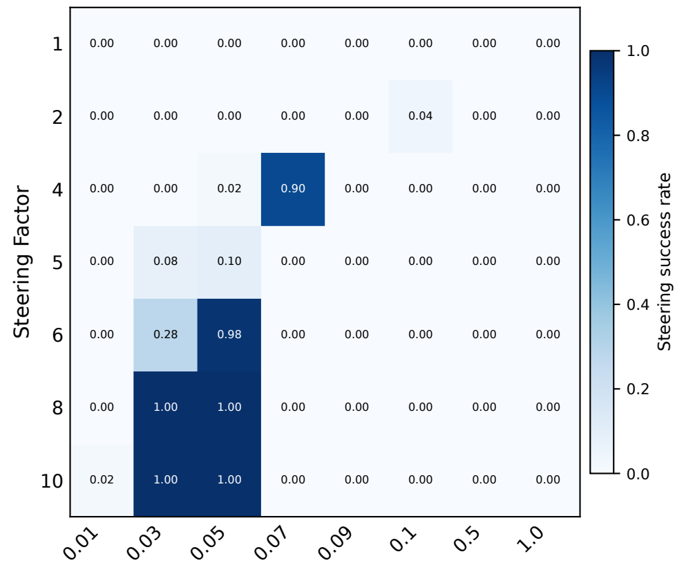
Qwen 1.5-14B
