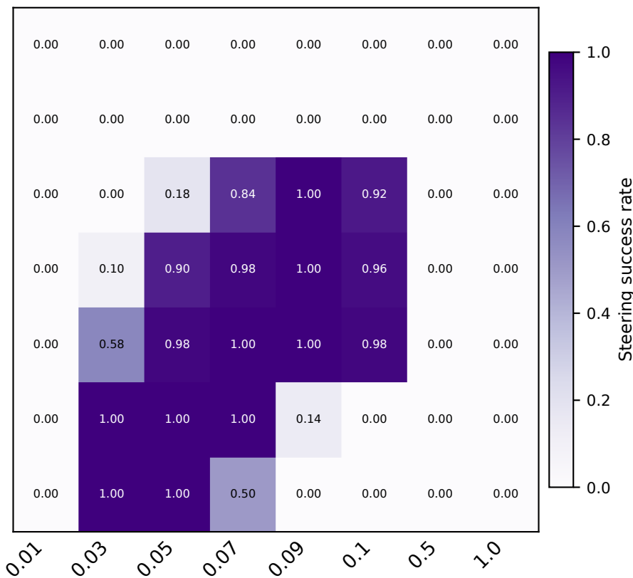
Qwen 1.5-32B
