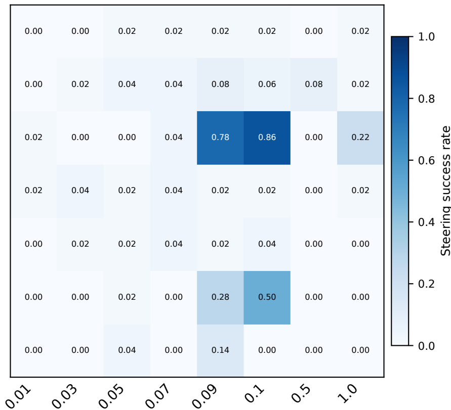
Qwen 1.5-14B
