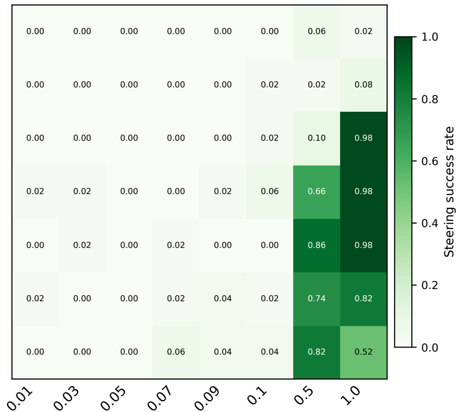
OLMo 2-13B
