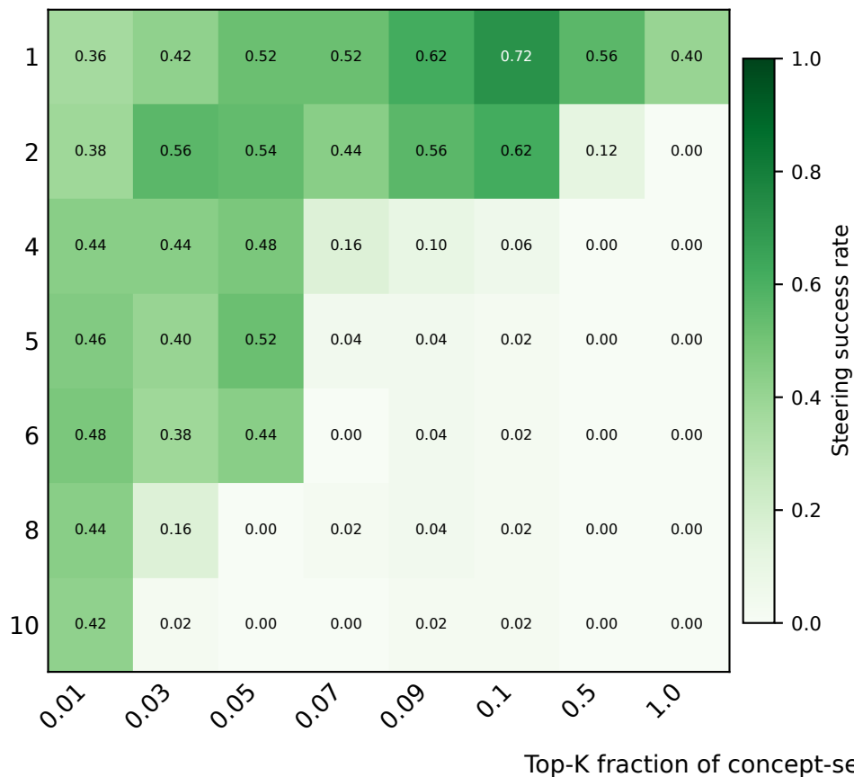
OLMo 2-13B
