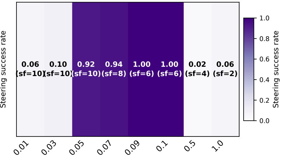
Qwen 1.5-32B
