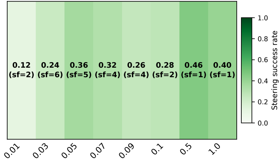
OLMo 2-13B
