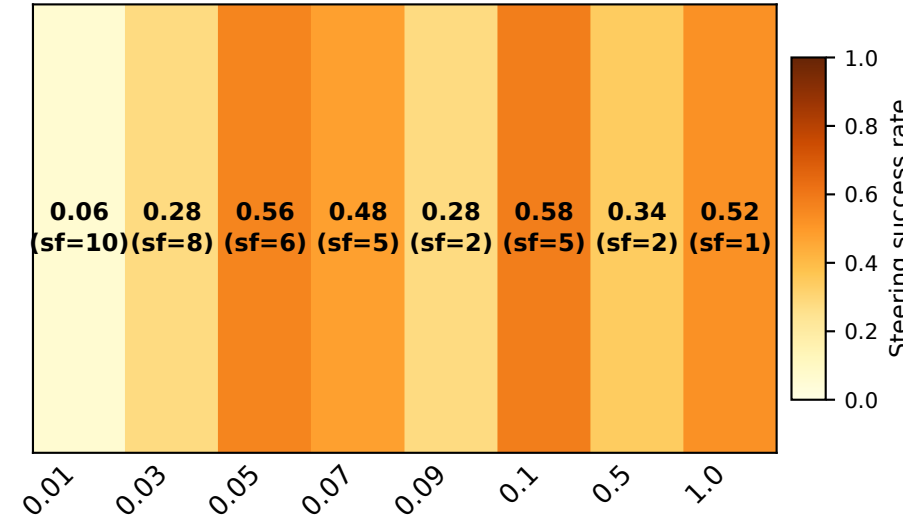
Gemma 3-12B
