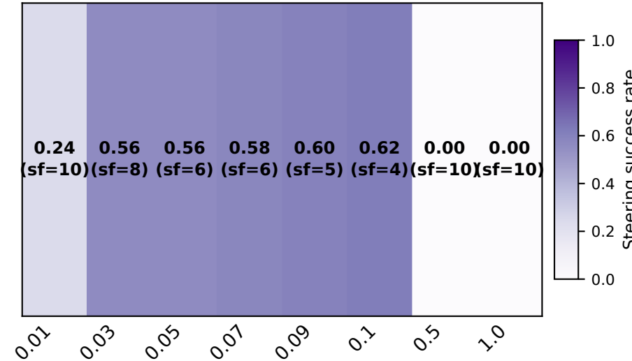
Qwen 1.5-32B
