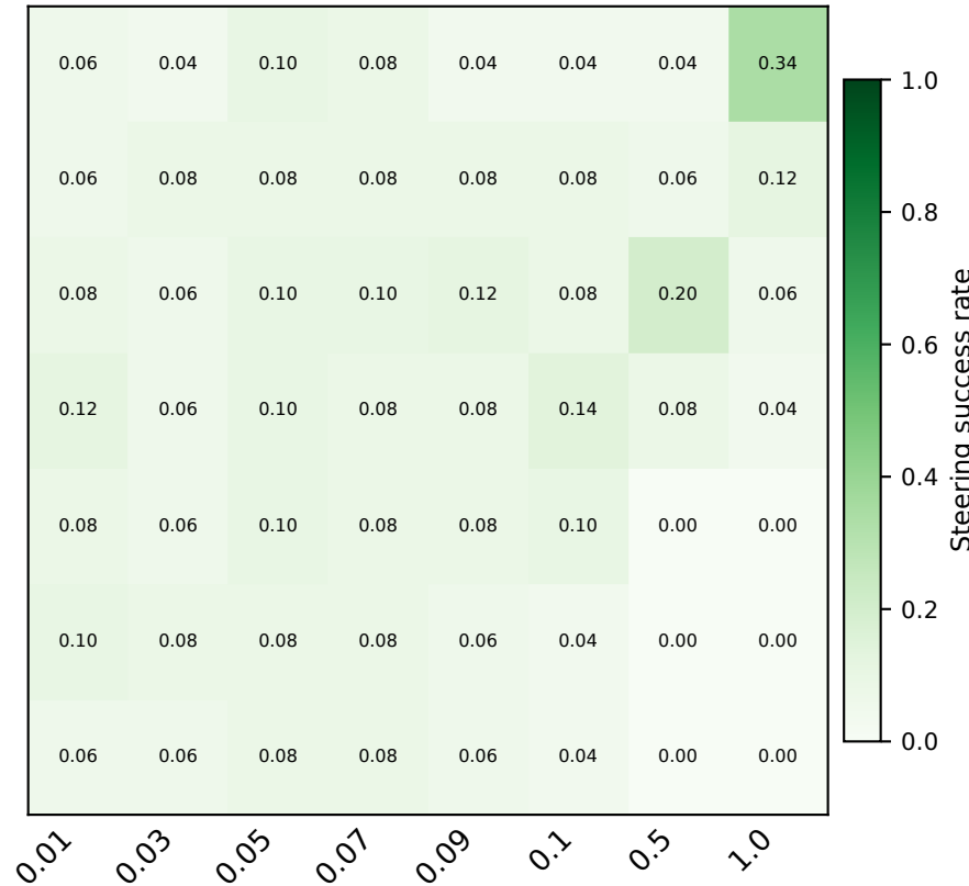
OLMo 2-13B
