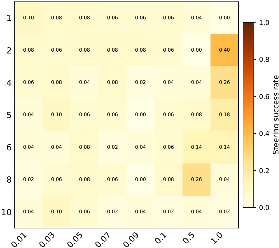
Gemma 3-12B
