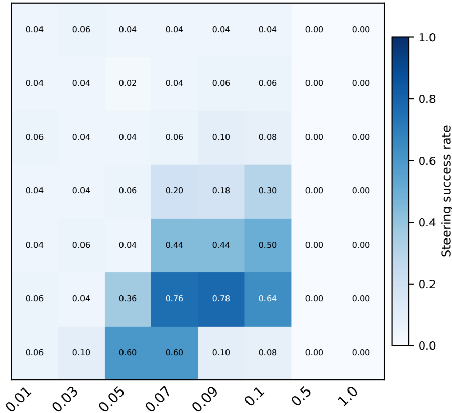
Qwen 1.5-14B
