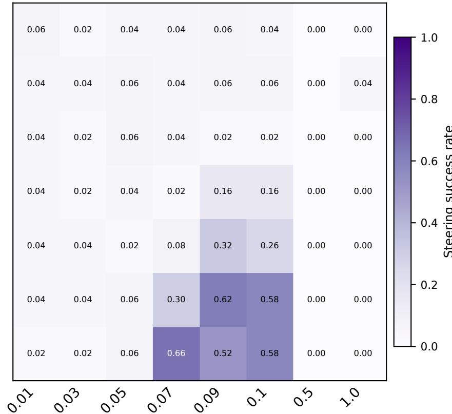
Qwen 1.5-32B
