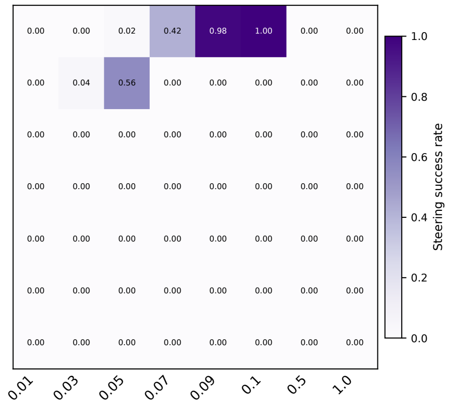
Vicuna 13B
