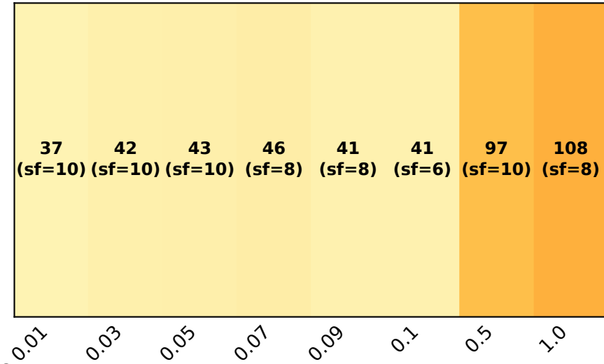
Gemma 3-12B
