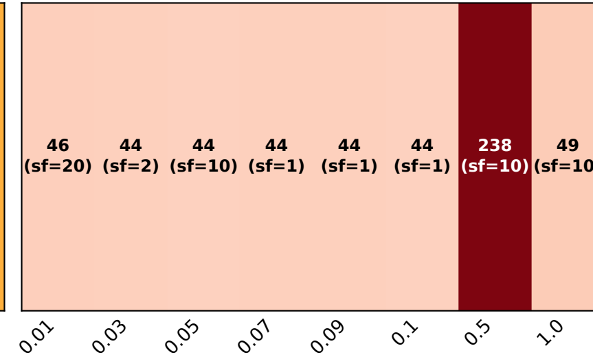
Falcon3-10B
