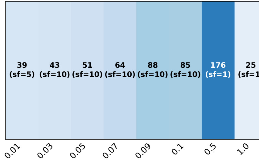
Qwen 1.5-14B
