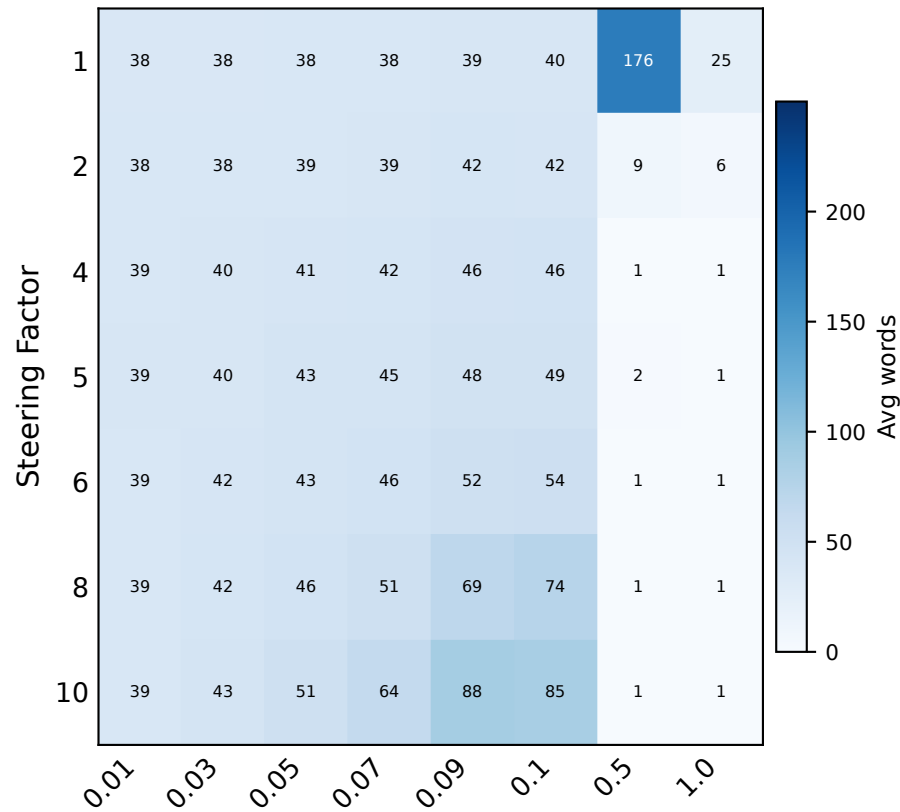
Qwen 1.5-14B
