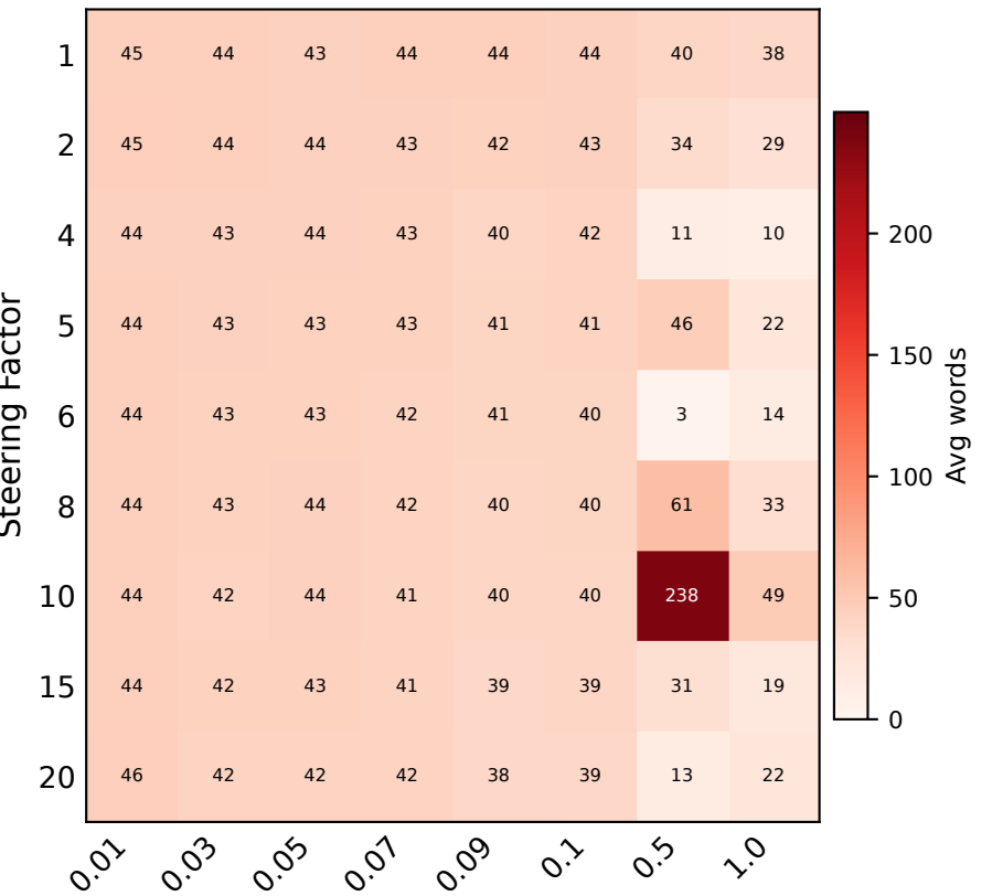
Falcon3-10B
