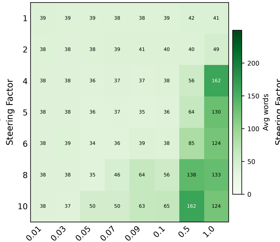
OLMo 2-13B
