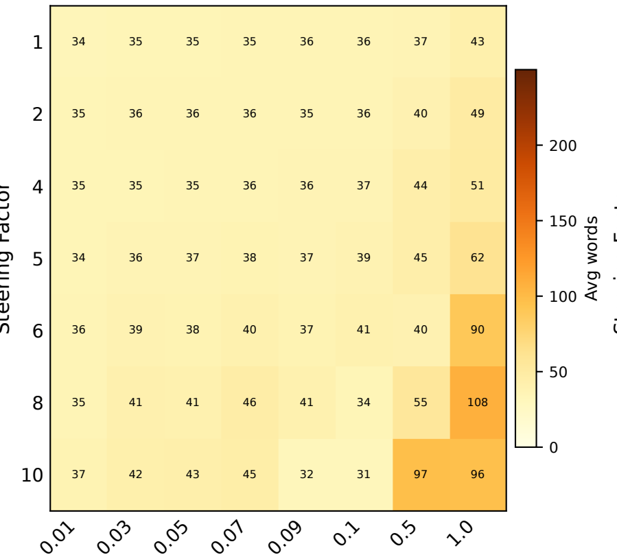
Gemma 3-12B
