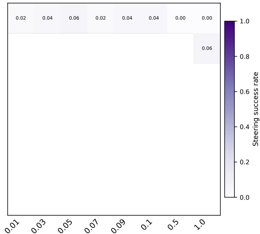
Qwen 1.5-32B
