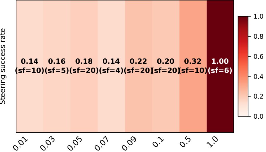
Falcon3-10B
