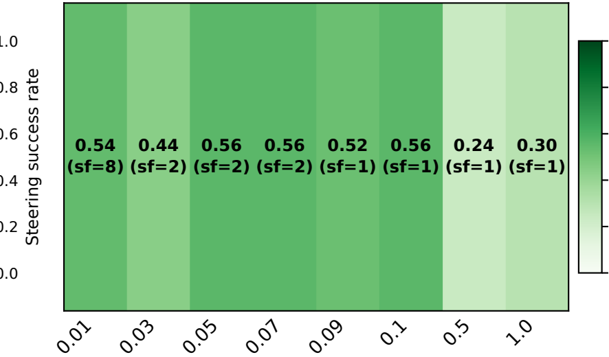
OLMo 2-13B
