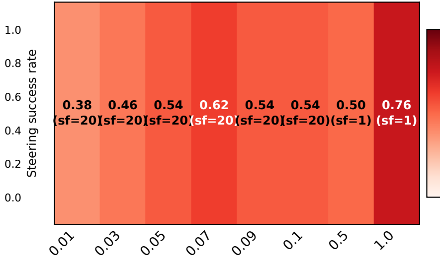
Falcon3-10B
