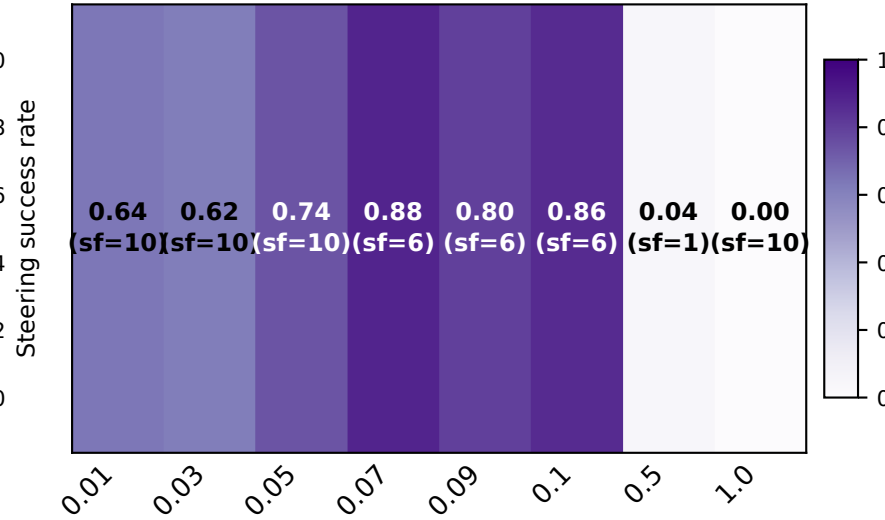
Qwen 1.5-32B
