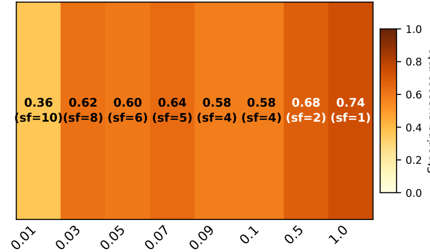
Gemma 3-12B
