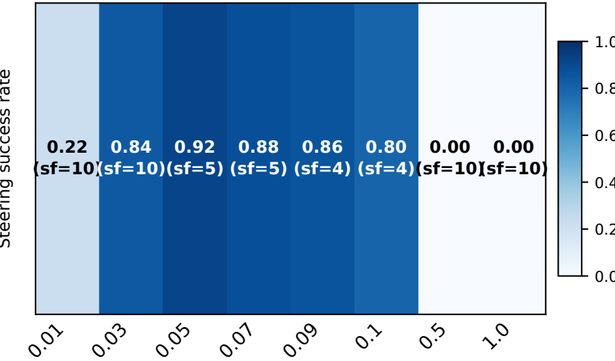
Qwen 1.5-14B
