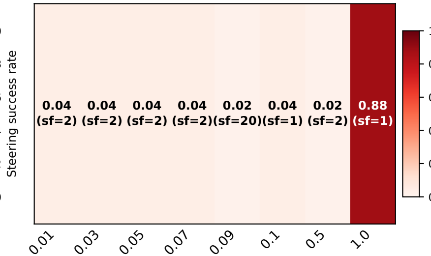
Falcon3-10B
