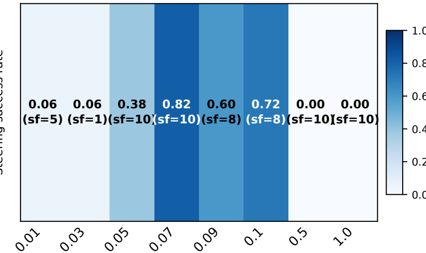
Qwen 1.5-14B
