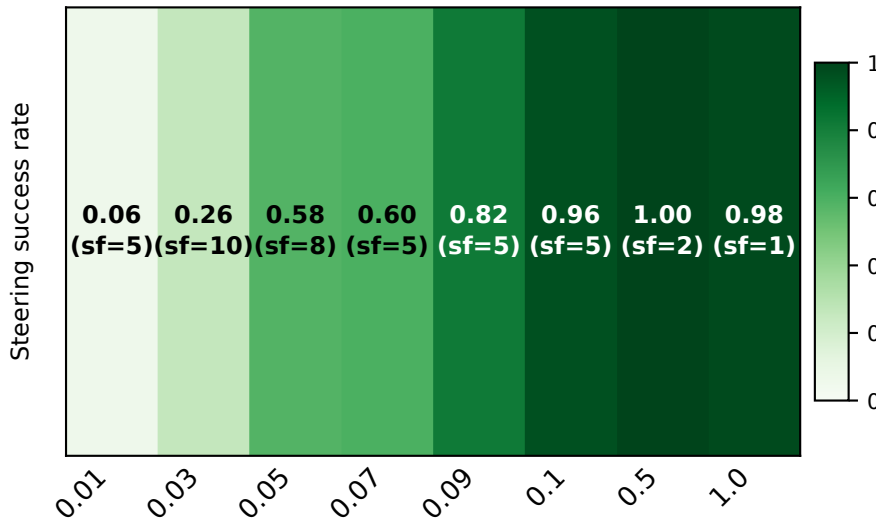
OLMo 2-13B
