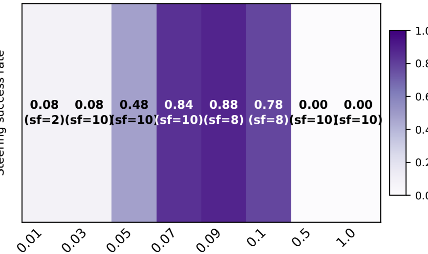
Qwen 1.5-32B
