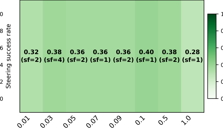
OLMo 2-13B
