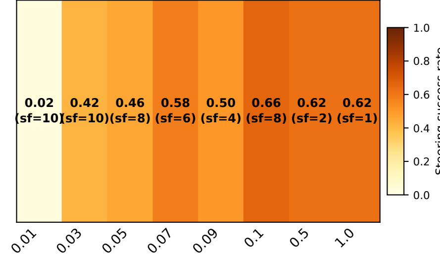
Gemma 3-12B
