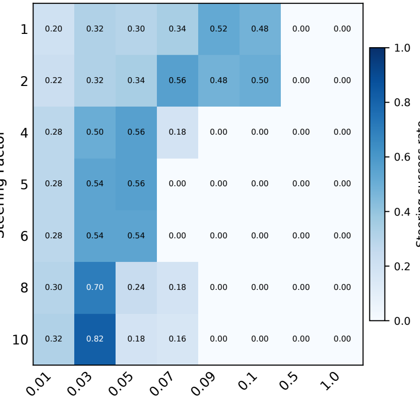
Qwen 1.5-14B
