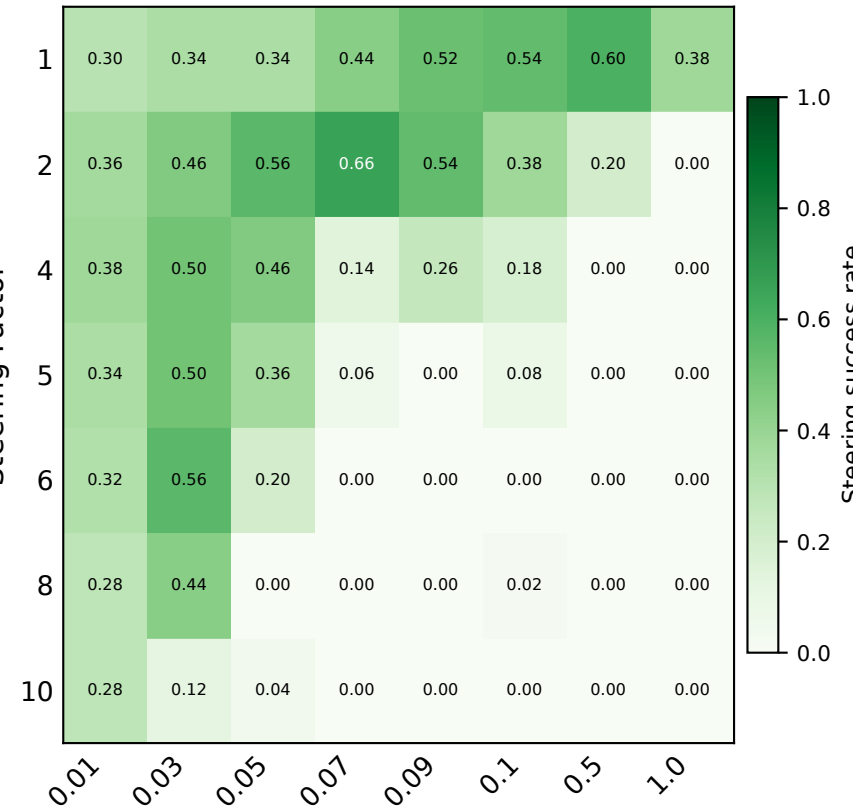
OLMo 2-13B
