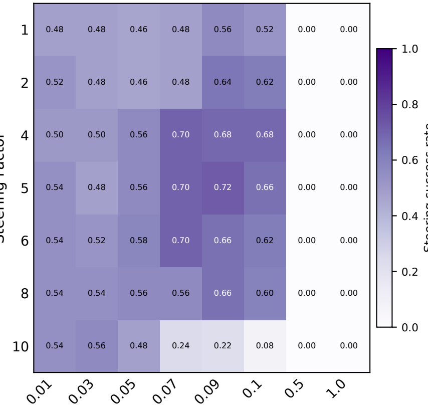
Qwen 1.5-32B
