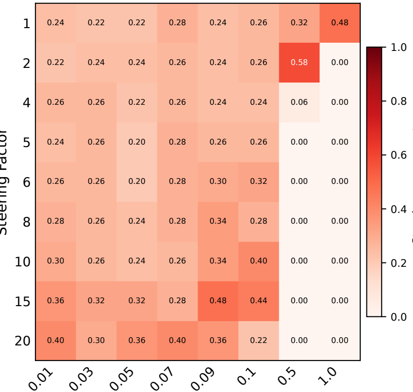
Falcon3-10B
