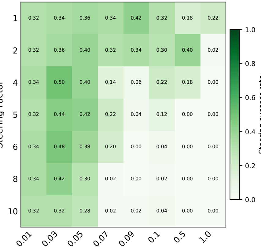
OLMo 2-13B
