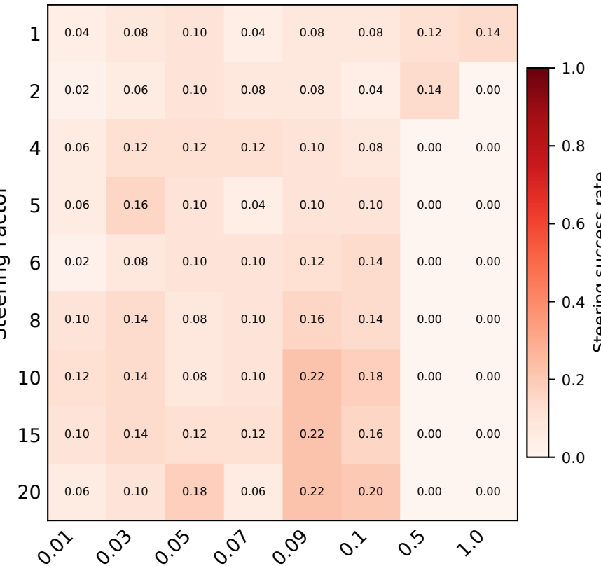
Falcon3-10B
