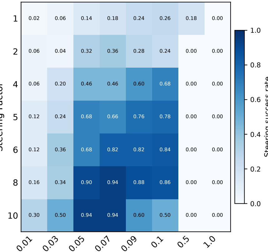
Qwen 1.5-14B
