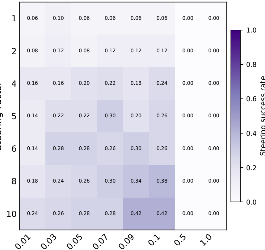
Qwen 1.5-32B
