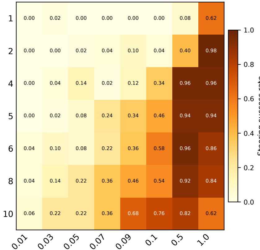
Gemma 3-12B
