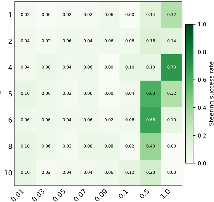
OLMo 2-13B
