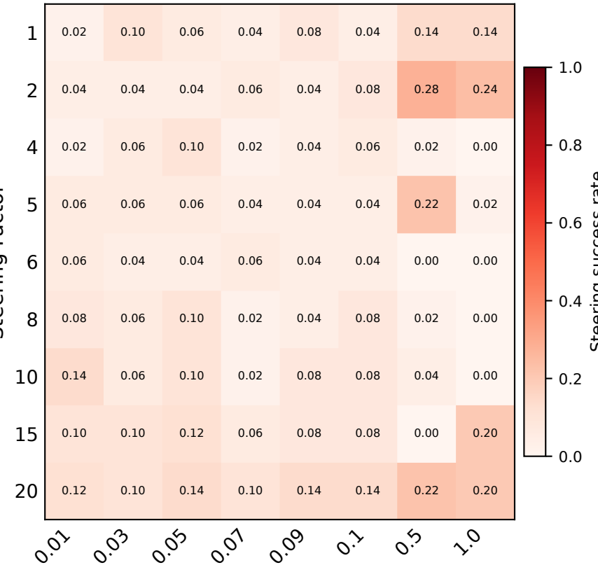
Falcon3-10B
