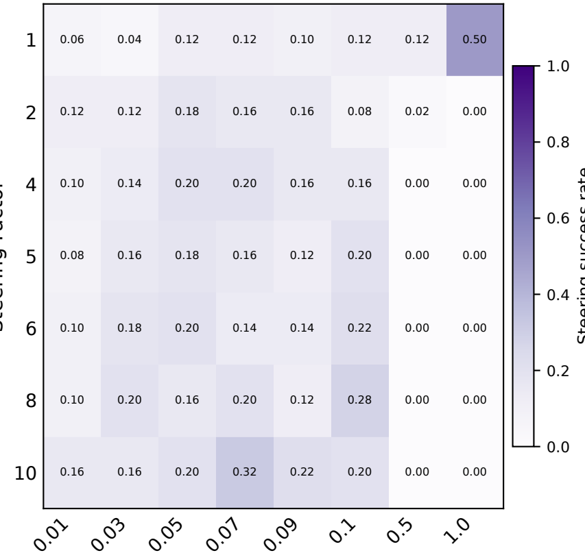
Qwen 1.5-32B
