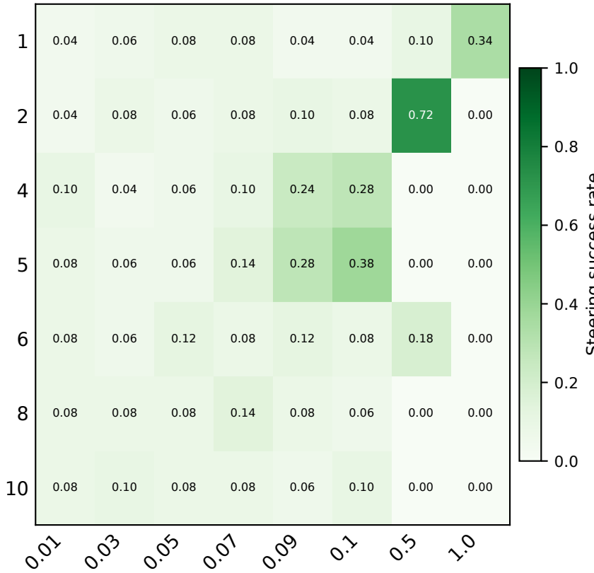
OLMo 2-13B
