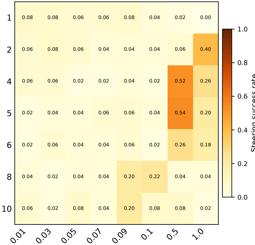
Gemma 3-12B
