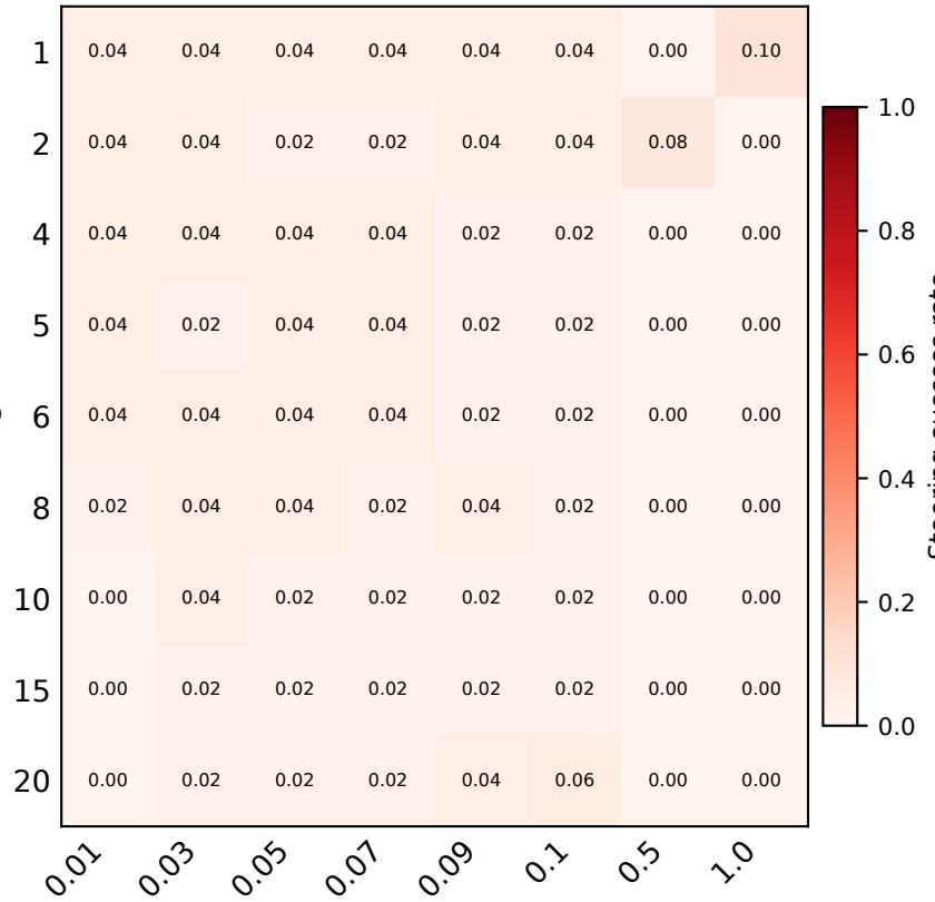
Falcon3-10B
