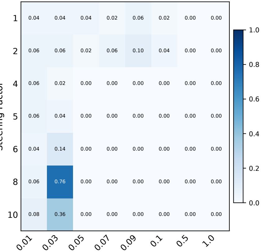
Qwen 1.5-14B
