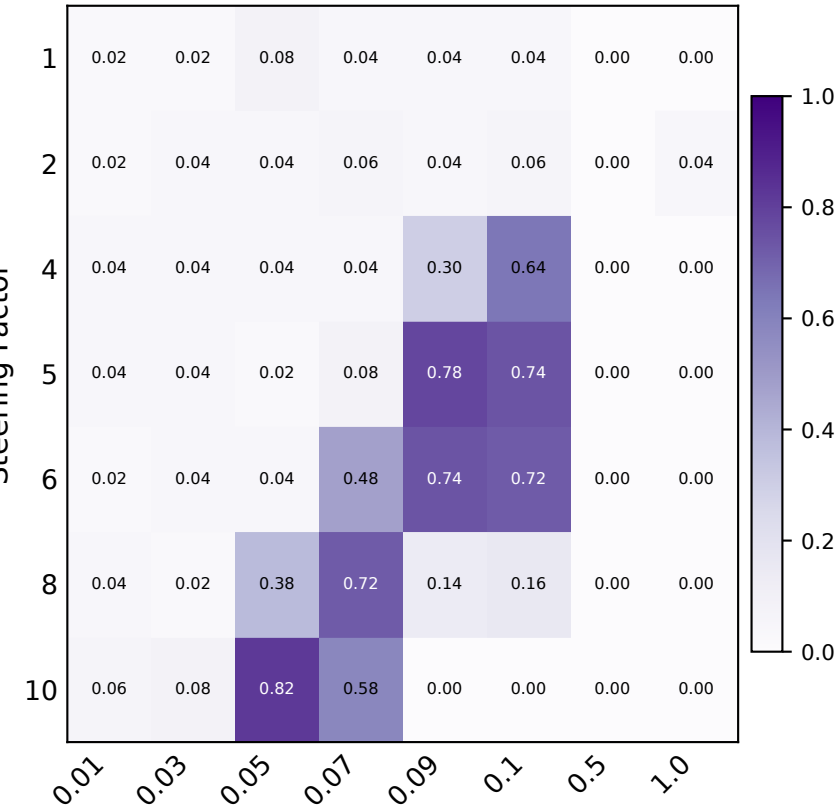
Qwen 1.5-32B
