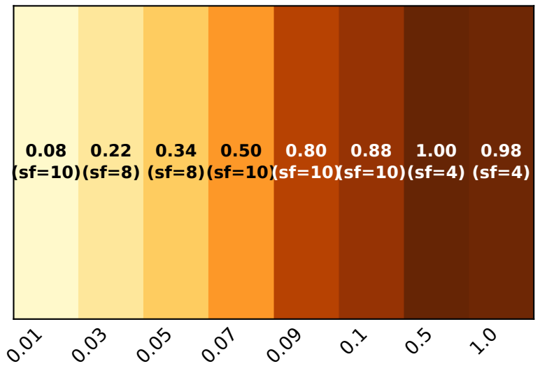
Gemma 3-12B
