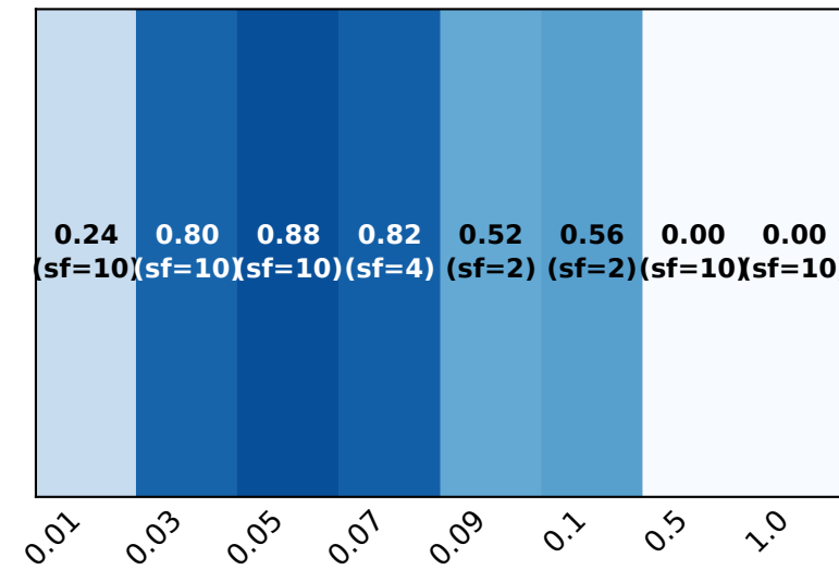
Qwen 1.5-14B
