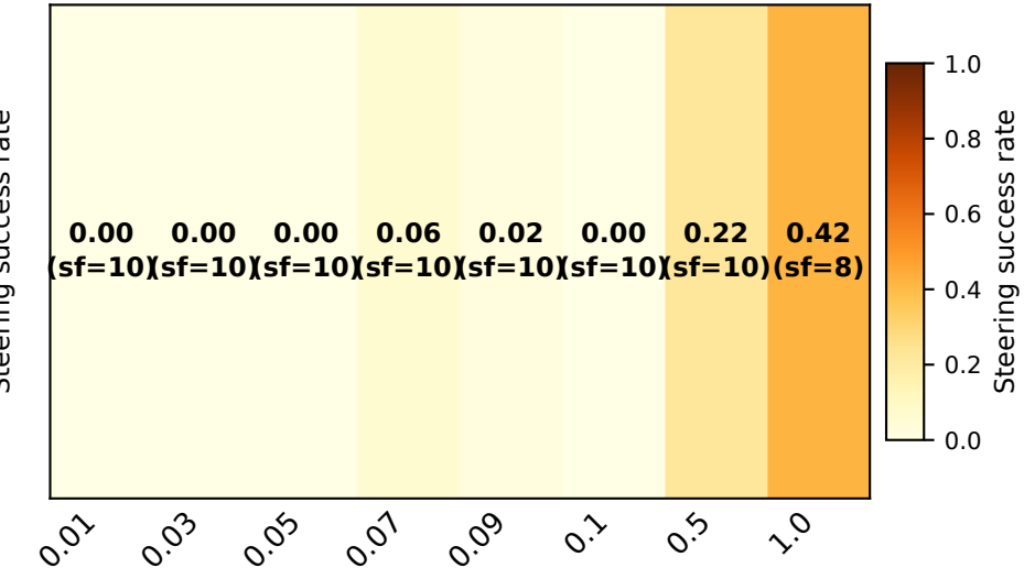
Gemma 3-12B
