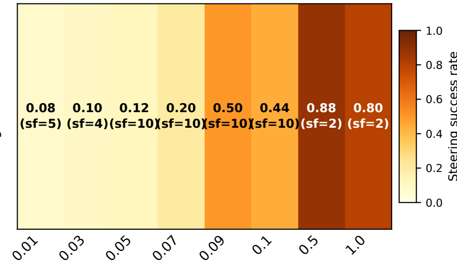
Gemma 3-12B
