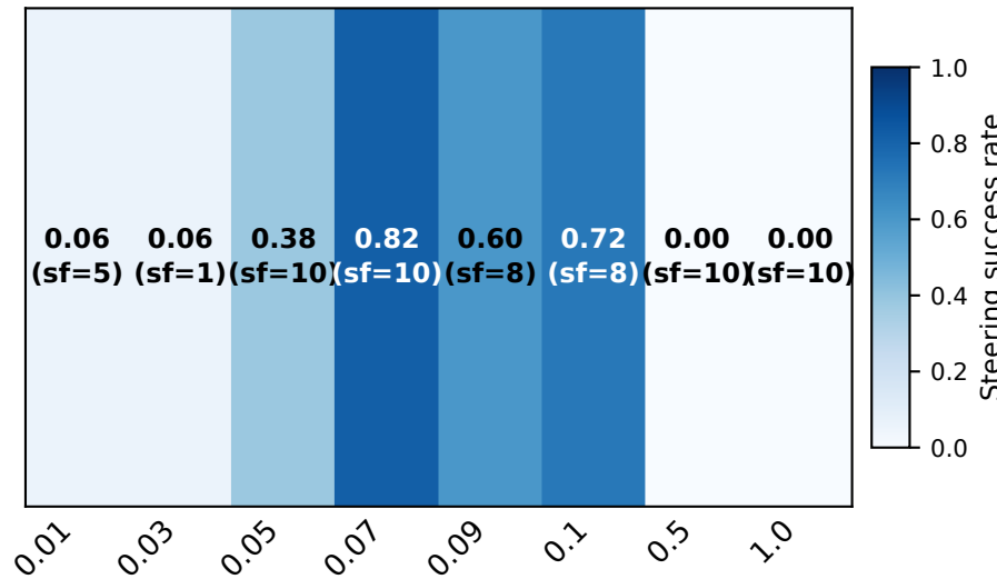
Qwen 1.5-14B
