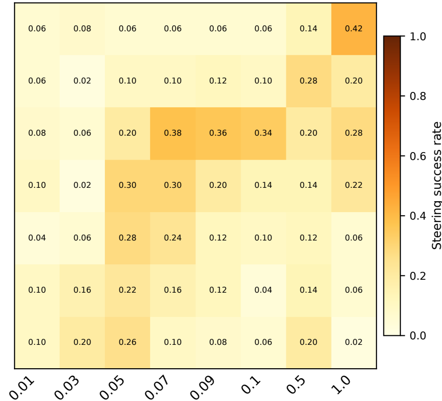
Gemma 3-12B
