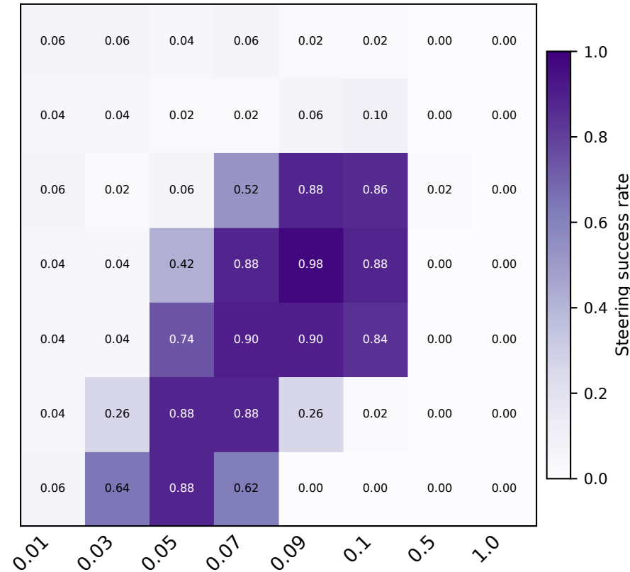
Qwen 1.5-32B
