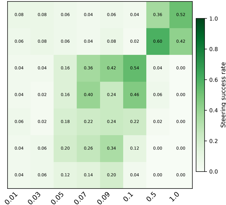
OLMo 2-13B
