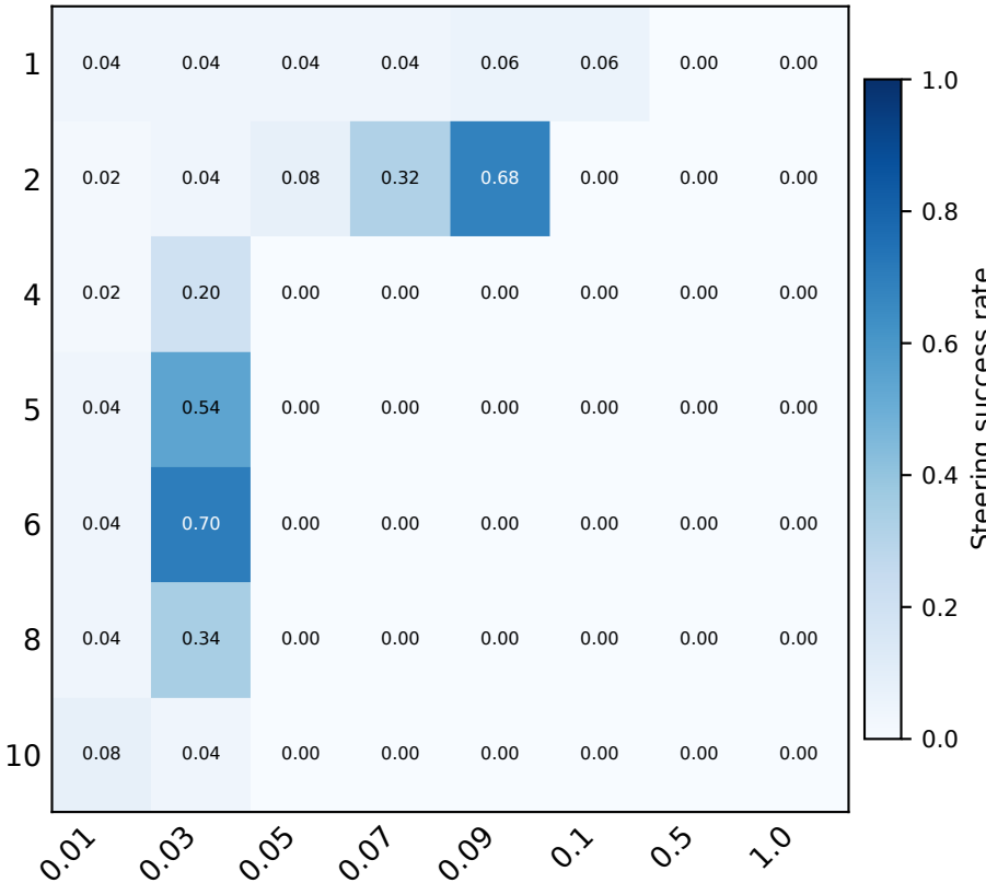
Qwen 1.5-14B
