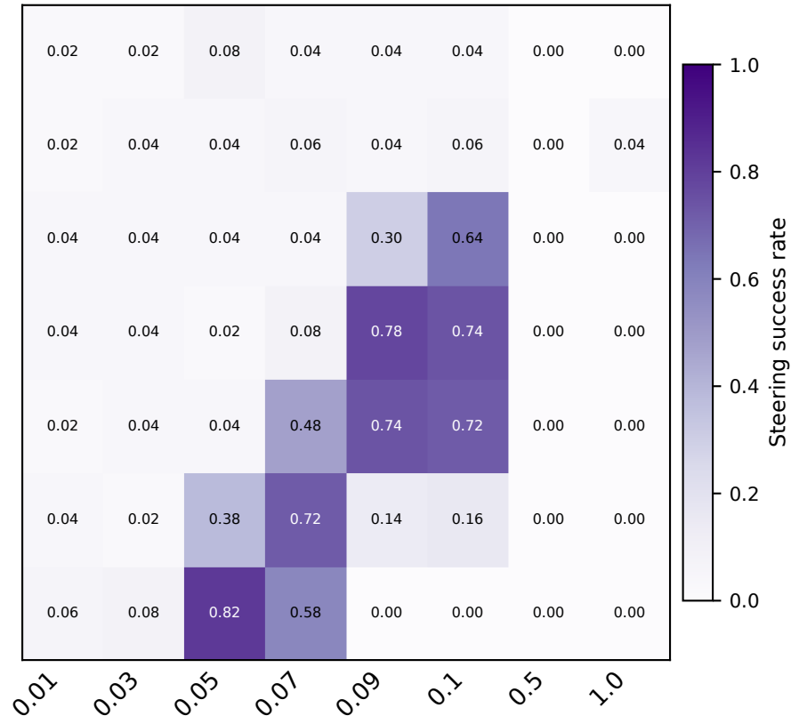
Qwen 1.5-32B
