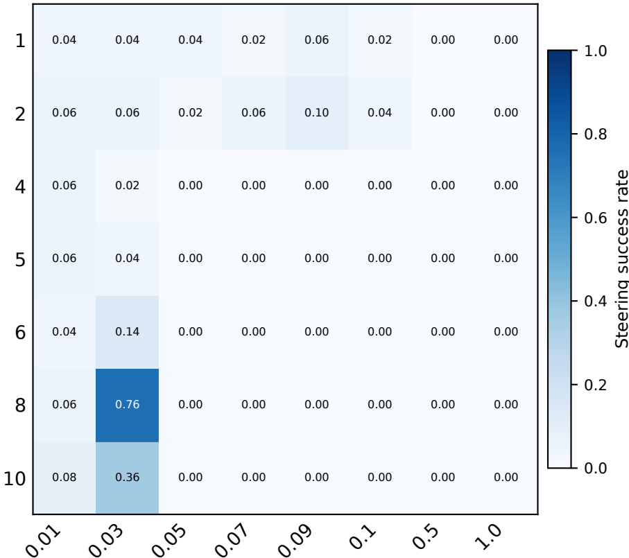
Qwen 1.5-14B
