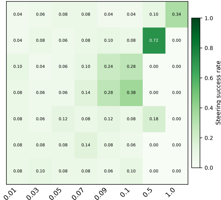
OLMo 2-13B
