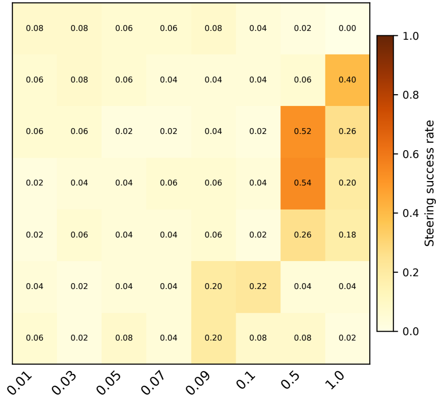
Gemma 3-12B
