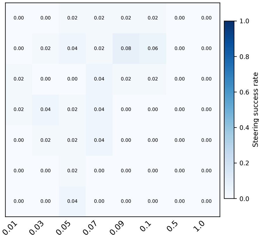
Qwen 1.5-14B
