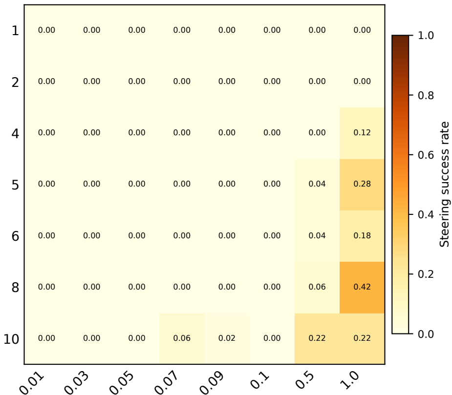
Gemma 3-12B
