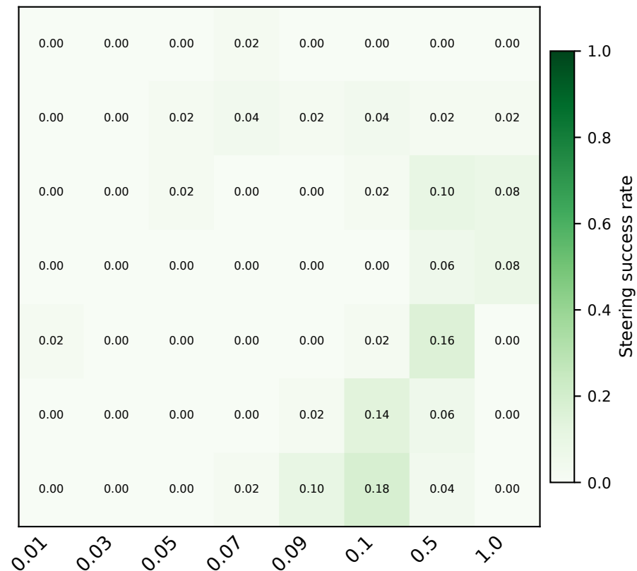
OLMo 2-13B
