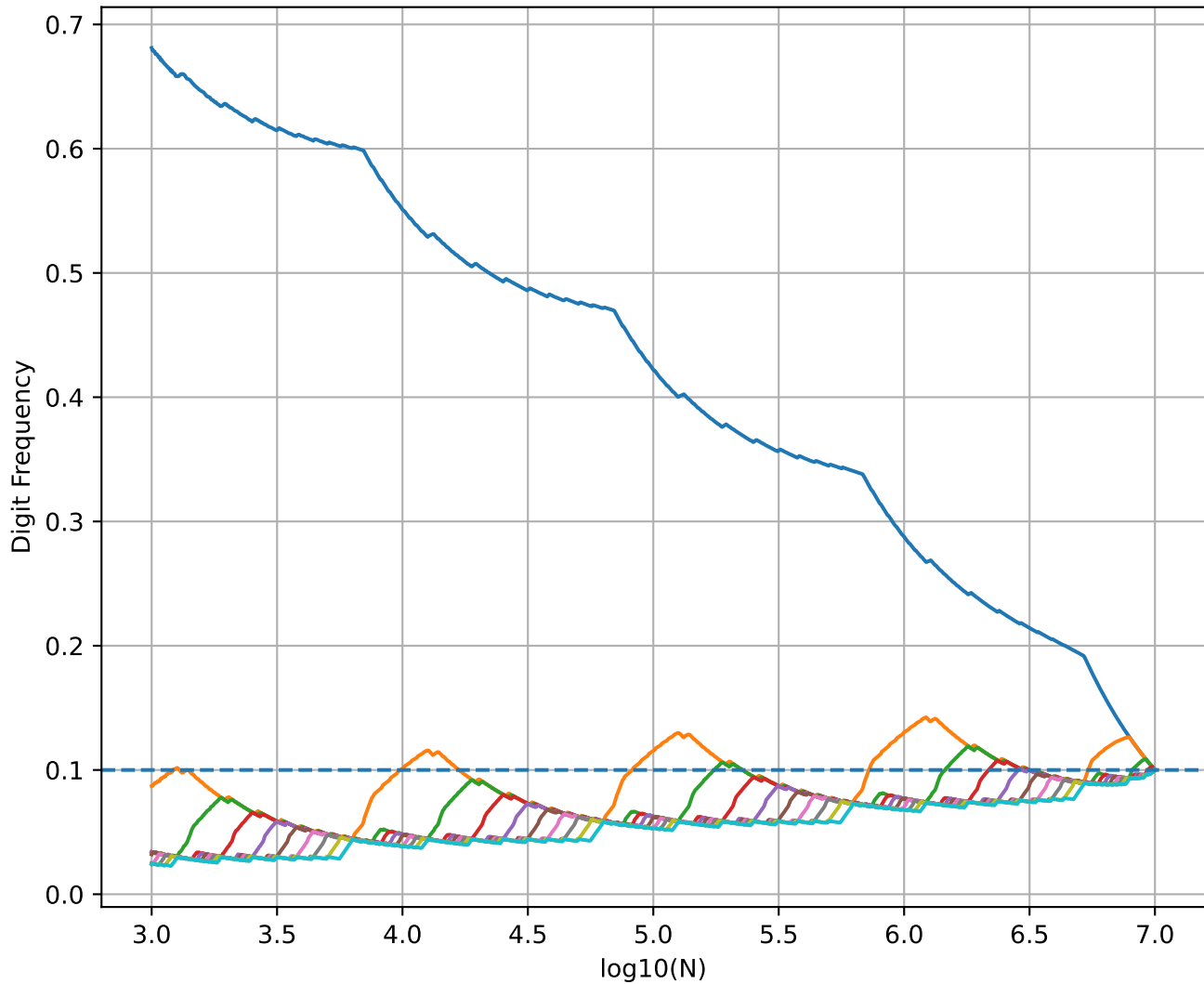
debruijn - Digit Convergence
