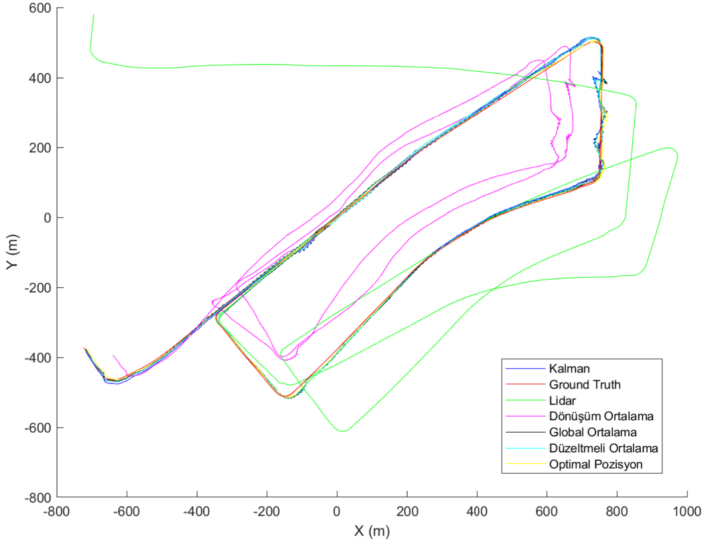
riverside3 Veriseti Kuş Bakışı Odometri Sonucu
