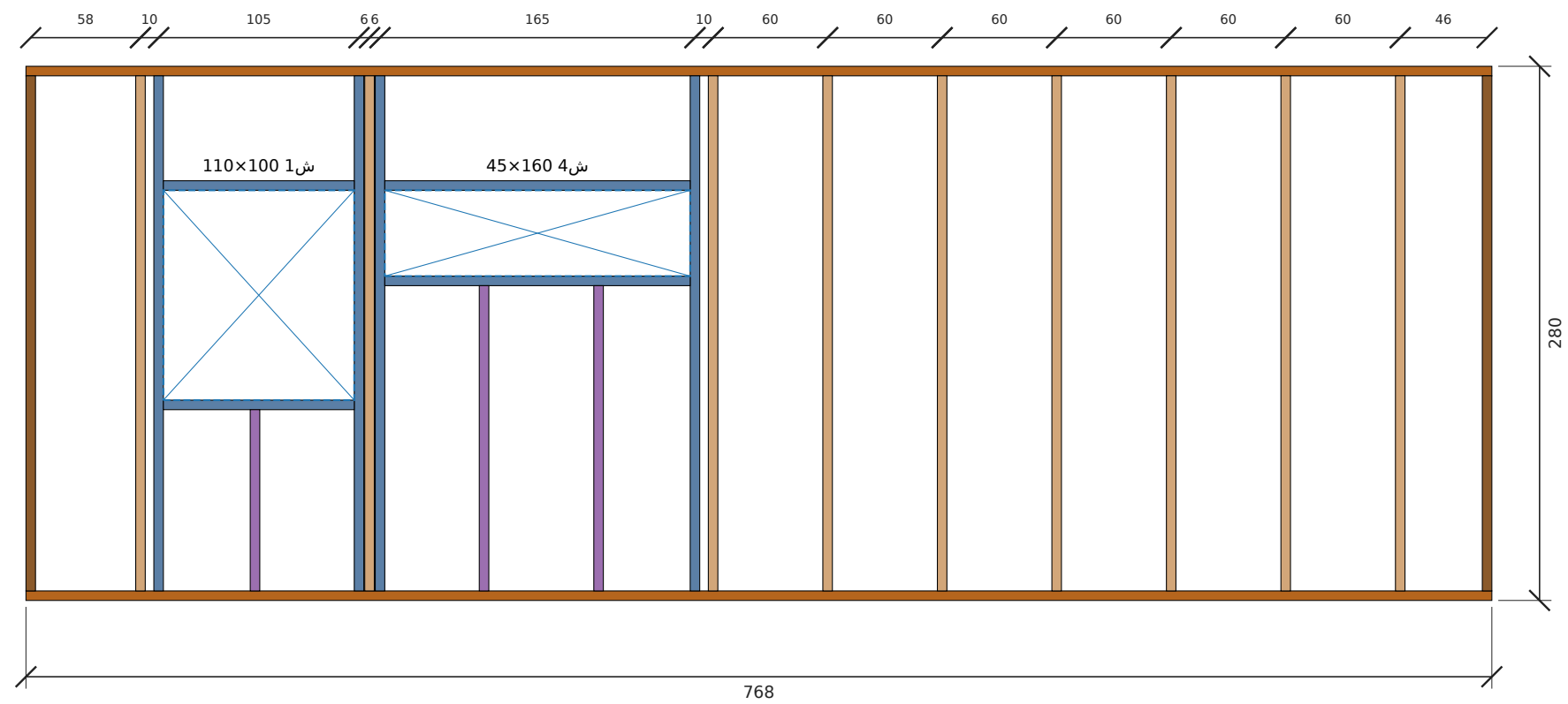
تأطير جدار غرب — الطول 768 سم، الارتفاع 280 سم
