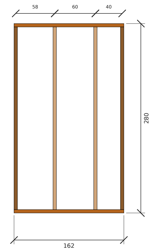
تأطير جدار د5-حمام ماستر جنوب — الطول 162 سم، الارتفاع 280 سم (داخلي)
