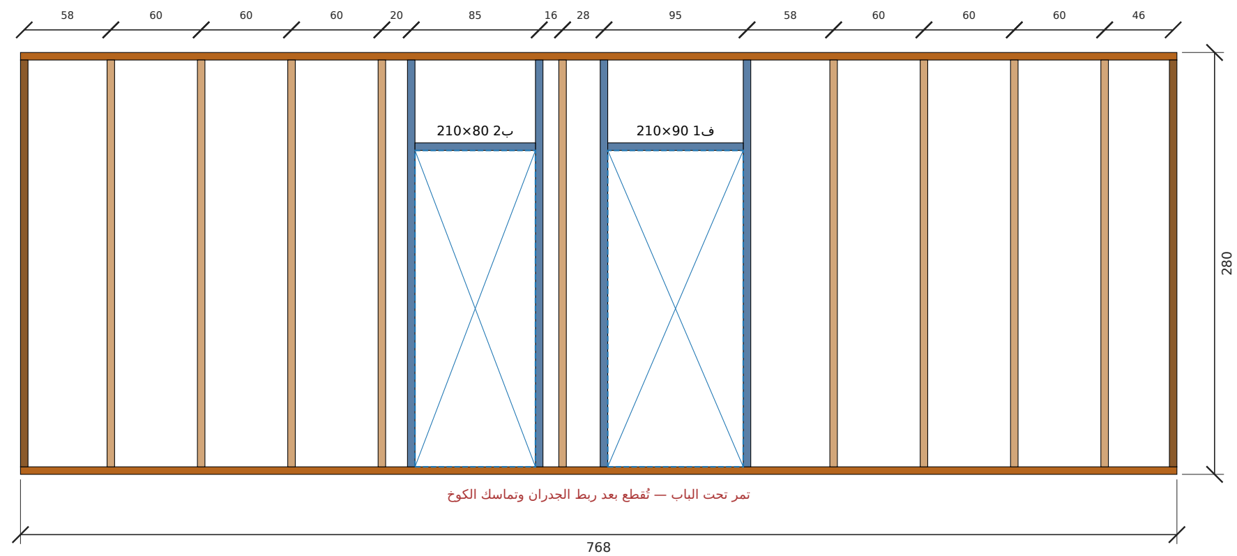
تأطير جدار د1-فاصل الصالة — الطول 768 سم، الارتفاع 280 سم (داخلي)
