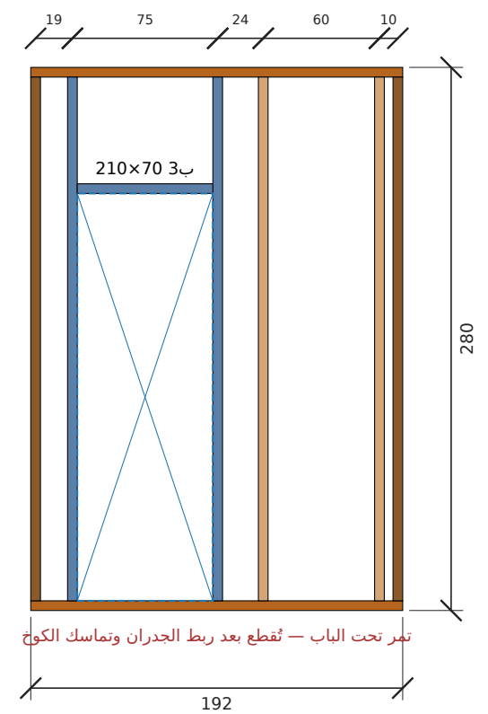
تأطير جدار د6-حمام ماستر غرب — الطول 192 سم، الارتفاع 280 سم (داخلي)
