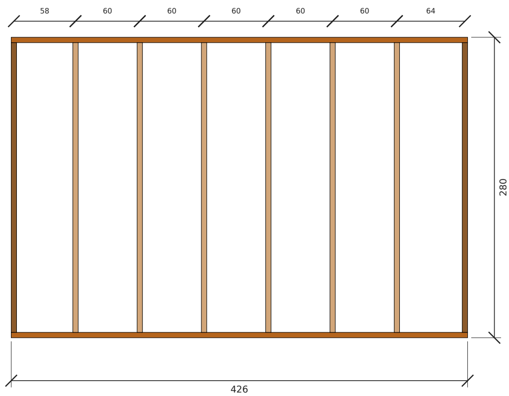
تأطير جدار د2-جدار النواة — الطول 426 سم، الارتفاع 280 سم (داخلي)
