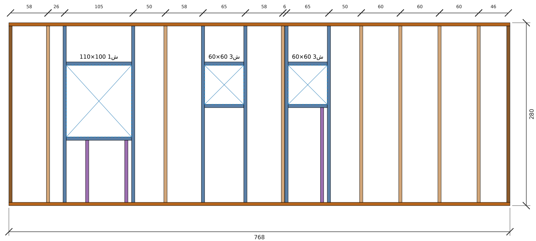
تأطير جدار شمال — الطول 768 سم، الارتفاع 280 سم
