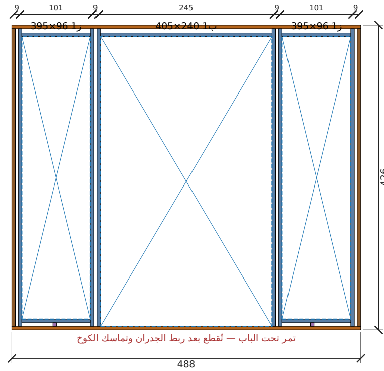
تأطير جدار جنوب — الطول 488 سم، الارتفاع 426 سم
