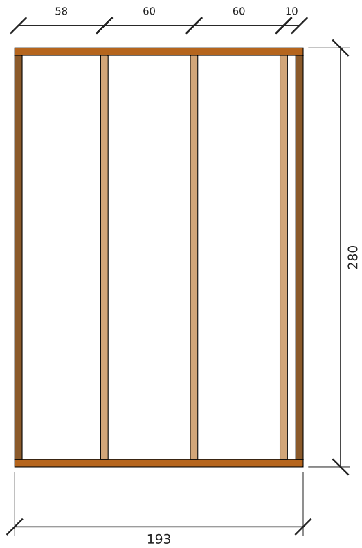
تأطير جدار د3-شرق حمام الصيوف — الطول 193 سم، الارتفاع 280 سم (داخلي)
