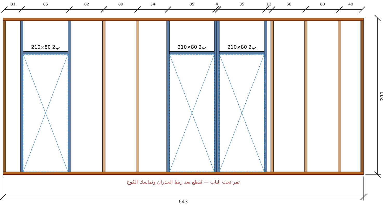
تأطير جدار د4-جنوب الغرف — الطول 643 سم، الارتفاع 280 سم (داخلي)
