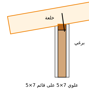
تفصيلة جلوس المداد على العلوي (1:5)
