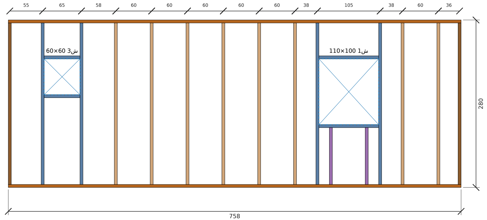
تأطير جدار ب-شرق — الطول 758 سم، الارتفاع 280 سم
