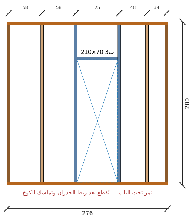
تأطير جدار ب-حمام الماستر — الطول 276 سم، الارتفاع 280 سم (داخلي)
