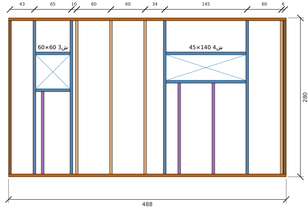
تأطير جدار شمال — الطول 488 سم، الارتفاع 280 سم
