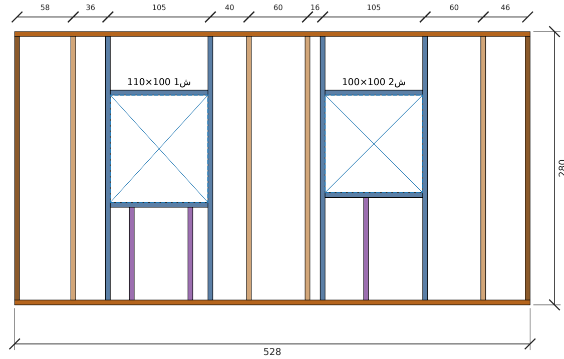
تأطير جدار غرب — الطول 528 سم، الارتفاع 280 سم
