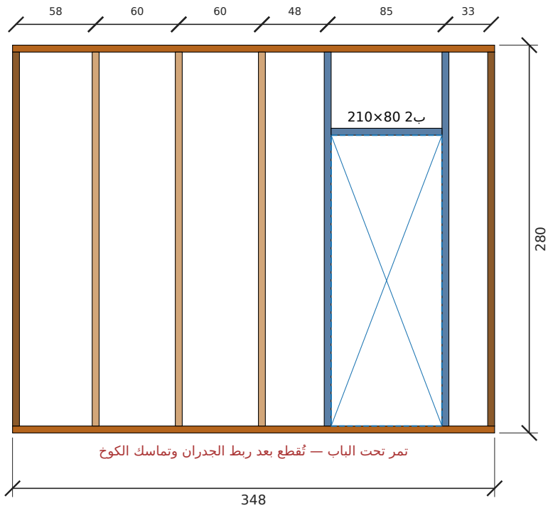
تأطير جدار ب-جدار الماستر — الطول 348 سم، الارتفاع 280 سم (داخلي)
