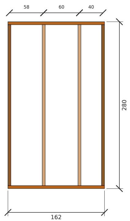
تأطير جدار أ-فاصل الحمامين — الطول 162 سم، الارتفاع 280 سم (داخلي)
