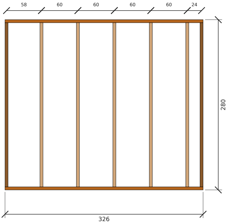
تأطير جدار ب-جدار الدرج — الطول 326 سم، الارتفاع 280 سم (داخلي)
