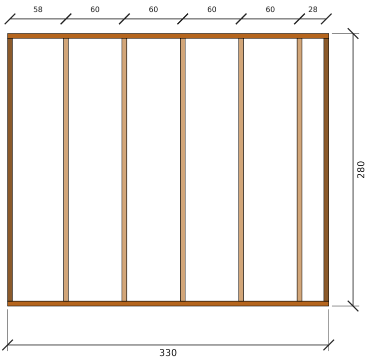
تأطير جدار ب-غرفة 2 شرق — الطول 330 سم، الارتفاع 280 سم (داخلي)
