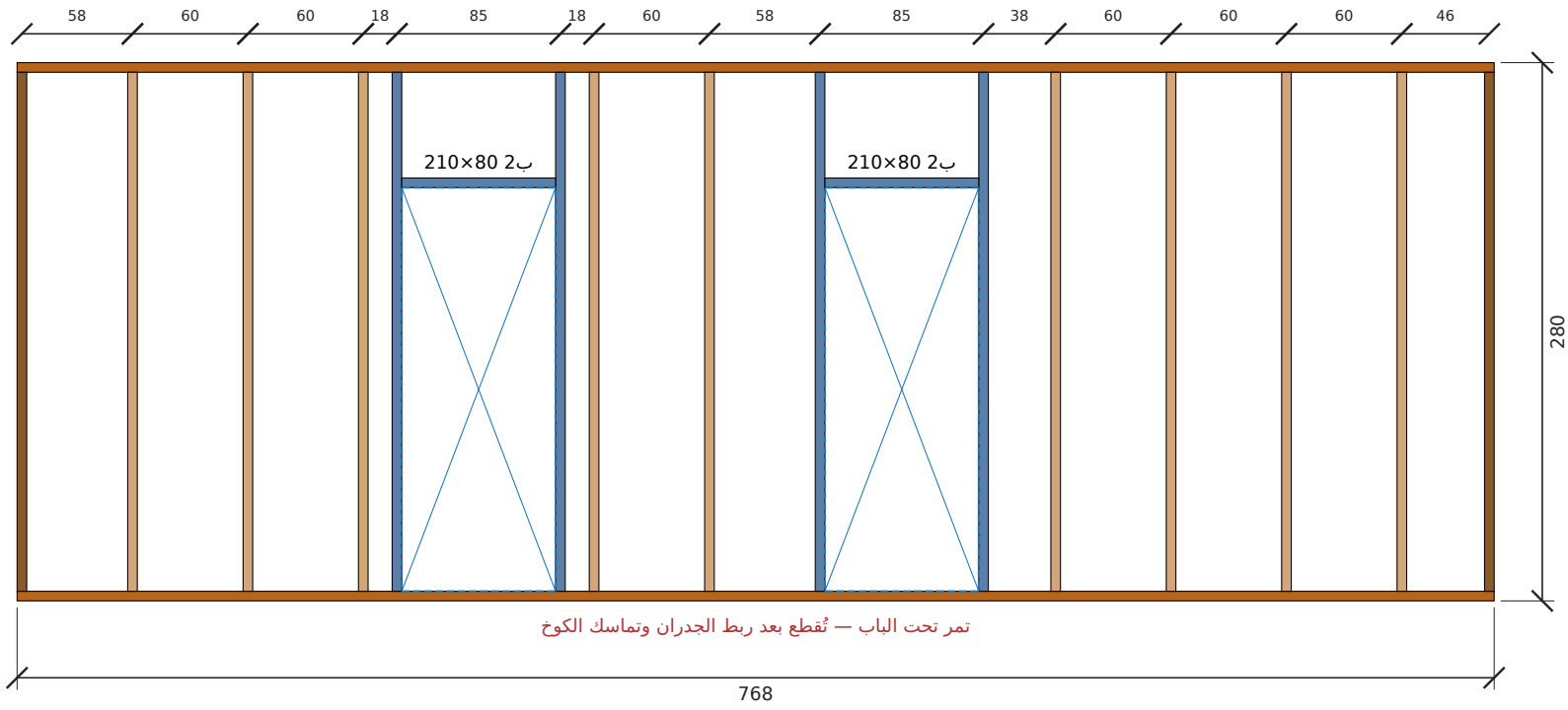
تأطير جدار ب-فاصل الغرف — الطول 768 سم، الارتفاع 280 سم (داخلي)
