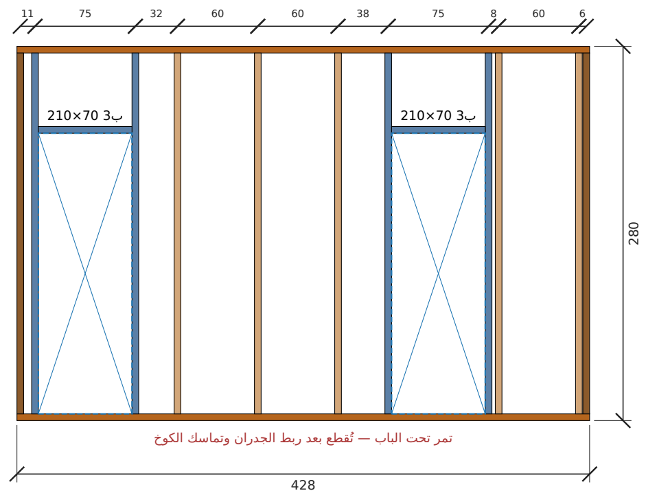
تأطير جدار أ-جدار الحمامات — الطول 428 سم، الارتفاع 280 سم (داخلي)
