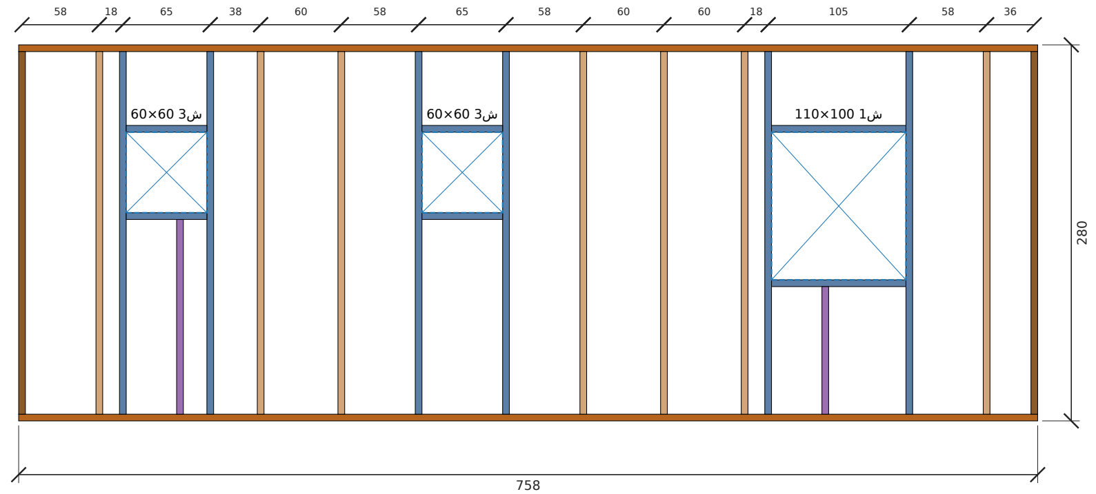
تأطير جدار ب-غرب — الطول 758 سم، الارتفاع 280 سم
