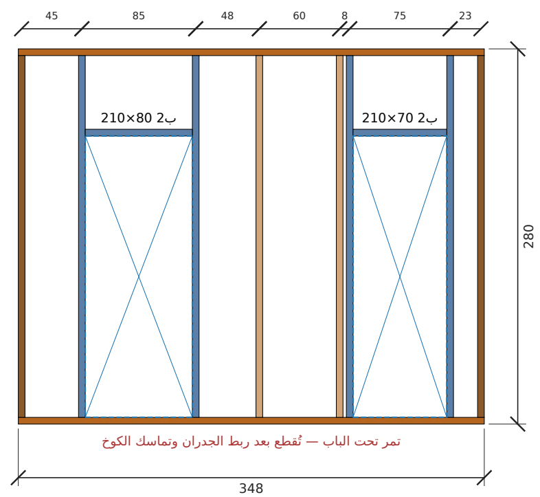
تأطير جدار أ-جدار الخادمة — الطول 348 سم، الارتفاع 280 سم (داخلي)
