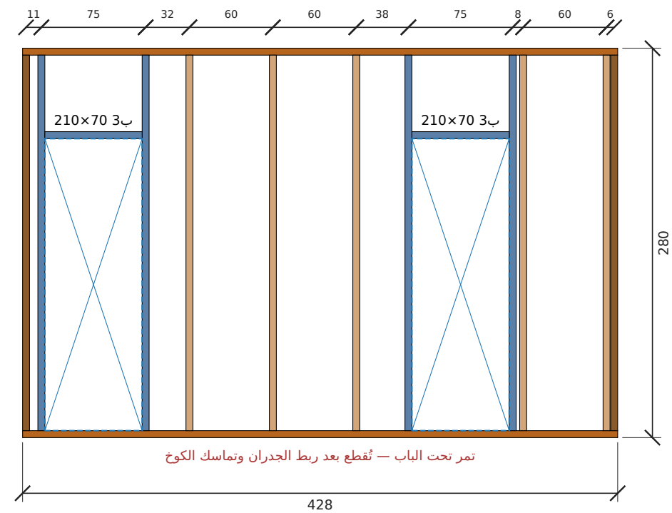
تأطير جدار ب-جدار الحمامات — الطول 428 سم، الارتفاع 280 سم (داخلي)
