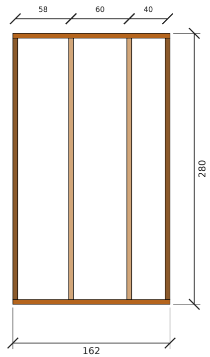
تأطير جدار ب-فاصل الحمامين — الطول 162 سم، الارتفاع 280 سم (داخلي)
