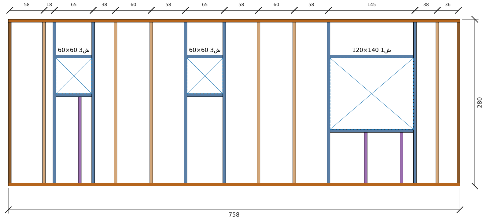
تأطير جدار أ-غرب — الطول 758 سم، الارتفاع 280 سم
