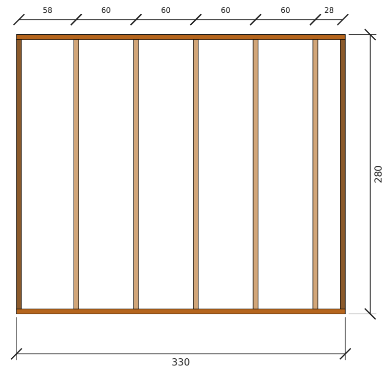
تأطير جدار أ-مطبخ غرب — الطول 330 سم، الارتفاع 280 سم (داخلي)
