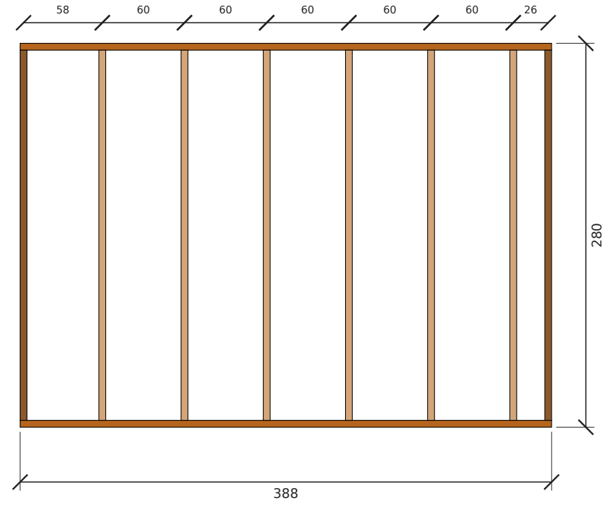
تأطير جدار شمال — الطول 388 سم، الارتفاع 280 سم
