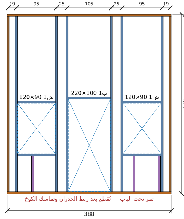
تأطير جدار جنوب — الطول 388 سم، الارتفاع 426 سم
