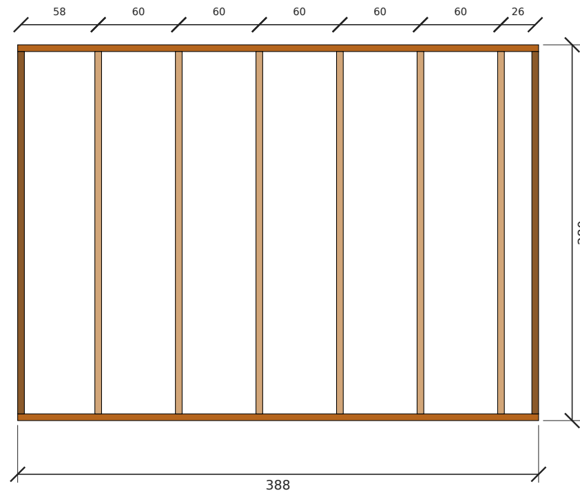
تأطير جدار شرق — الطول 388 سم، الارتفاع 280 سم
