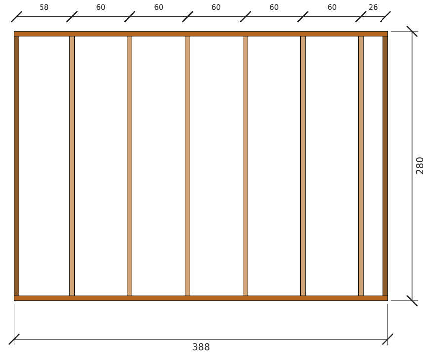
تأطير جدار غرب — الطول 388 سم، الارتفاع 280 سم
