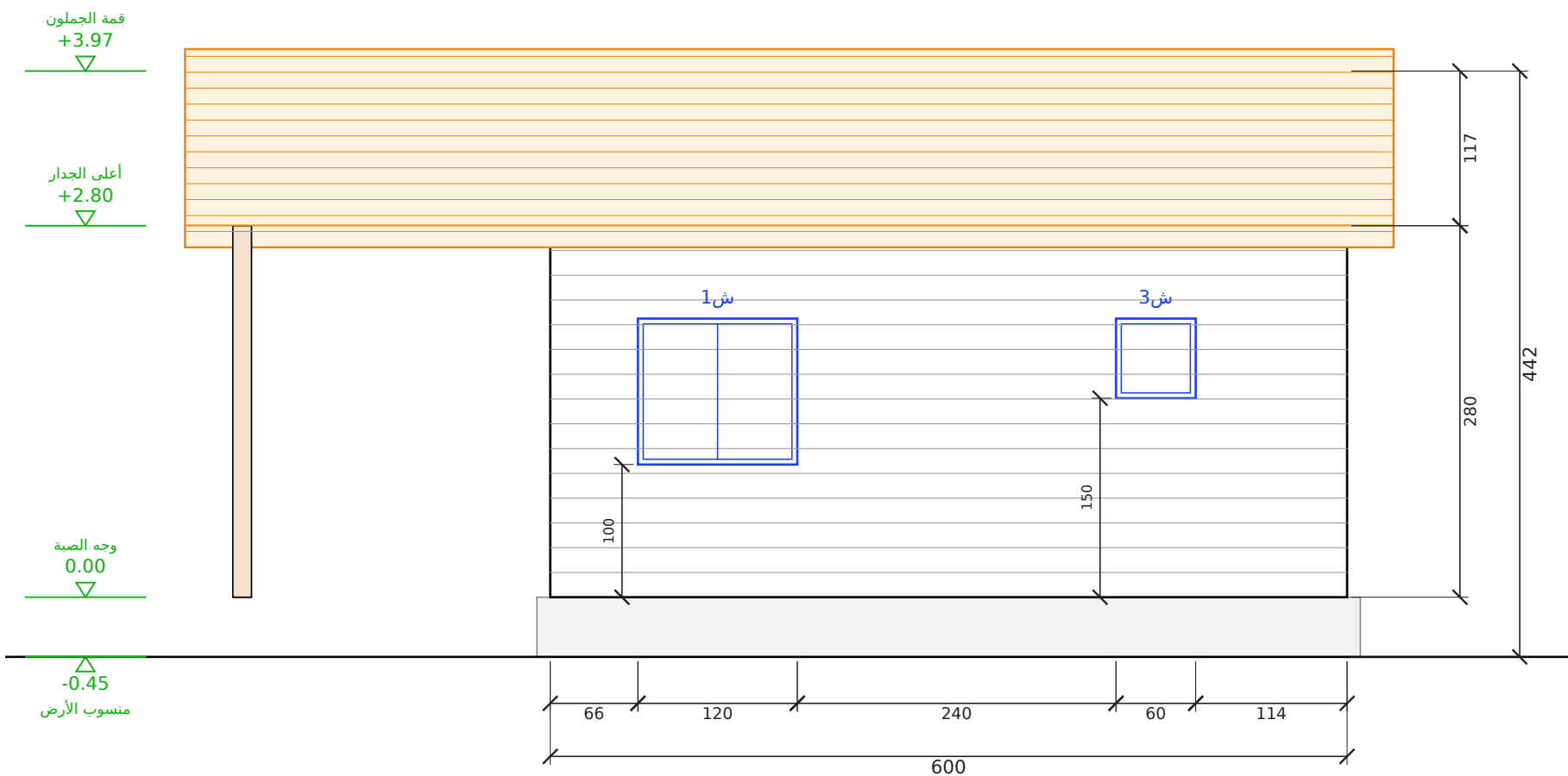
الواجهة الشرقية
