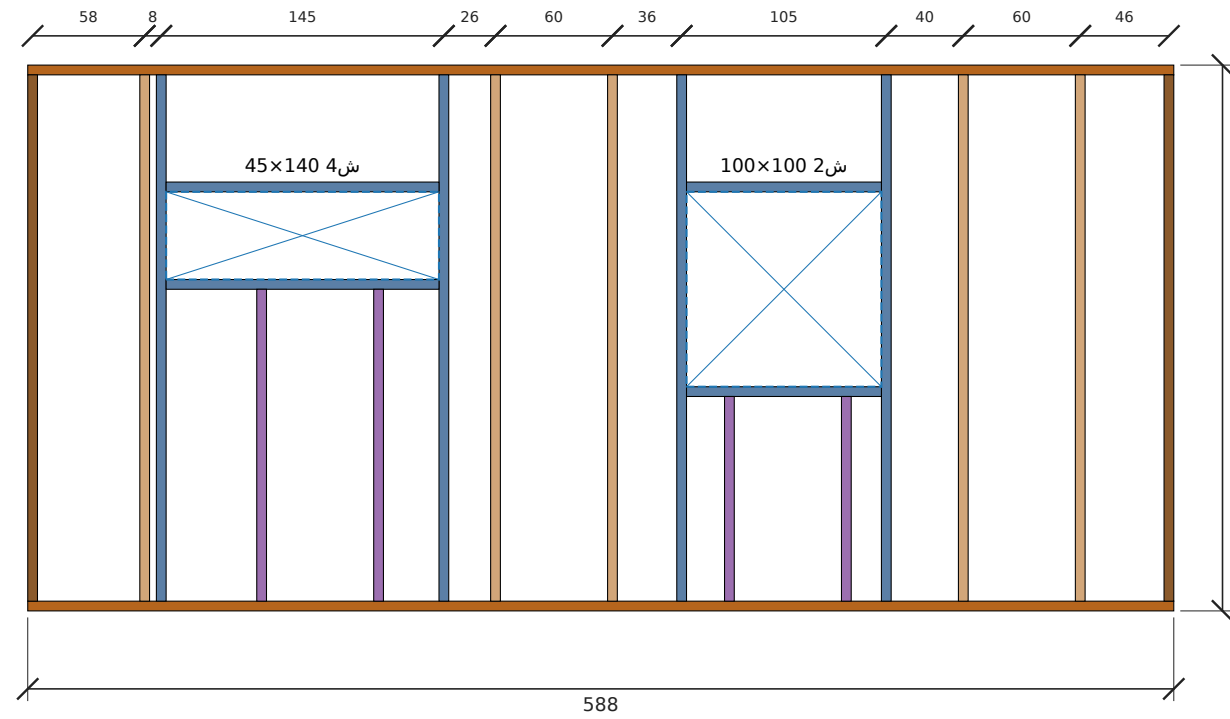
تأطير جدار غرب — الطول 588 سم، الارتفاع 280 سم
