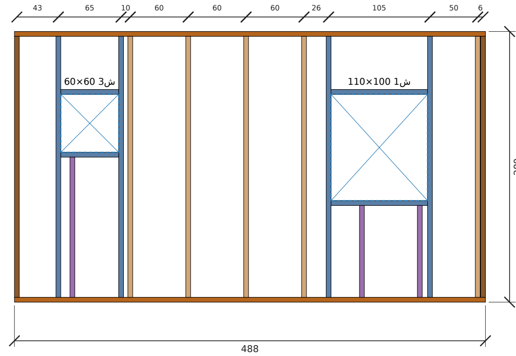
تأطير جدار شمال — الطول 488 سم، الارتفاع 280 سم
