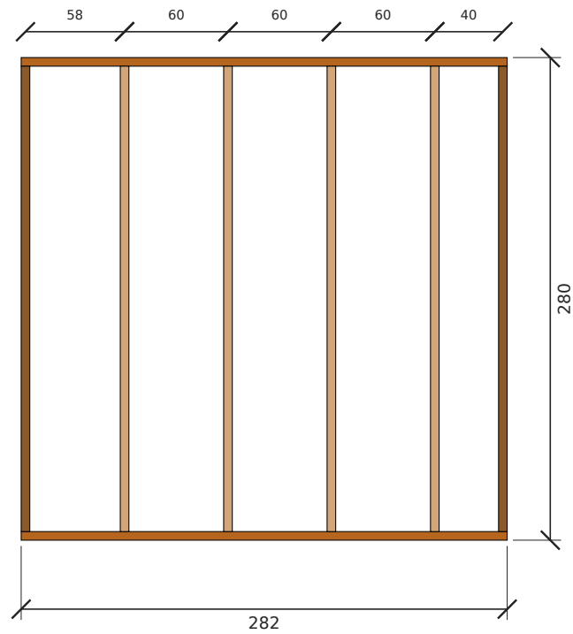
تأطير جدار د2-جدار الحمام — الطول 282 سم، الارتفاع 280 سم (داخلي)
