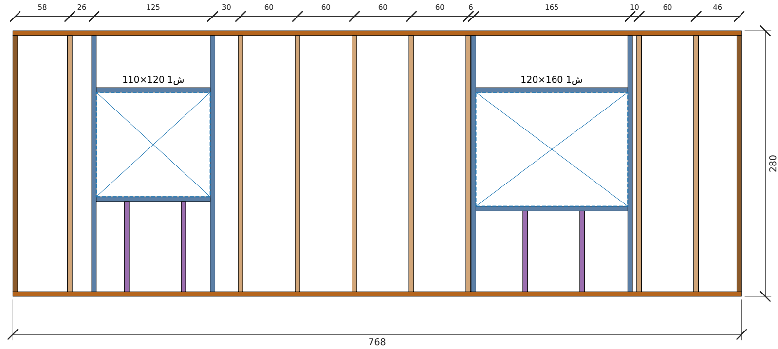
تأطير جدار أ-غرب — الطول 768 سم، الارتفاع 280 سم
