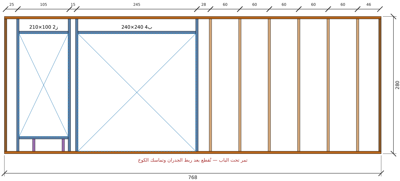
تأطير جدار ب-جنوب — الطول 768 سم، الارتفاع 280 سم
