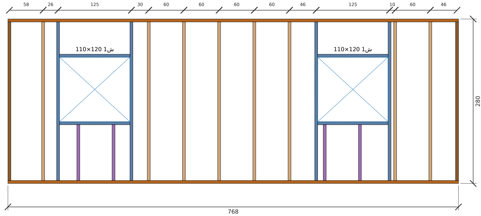
تأطير جدار ب-غرب — الطول 768 سم، الارتفاع 280 سم
