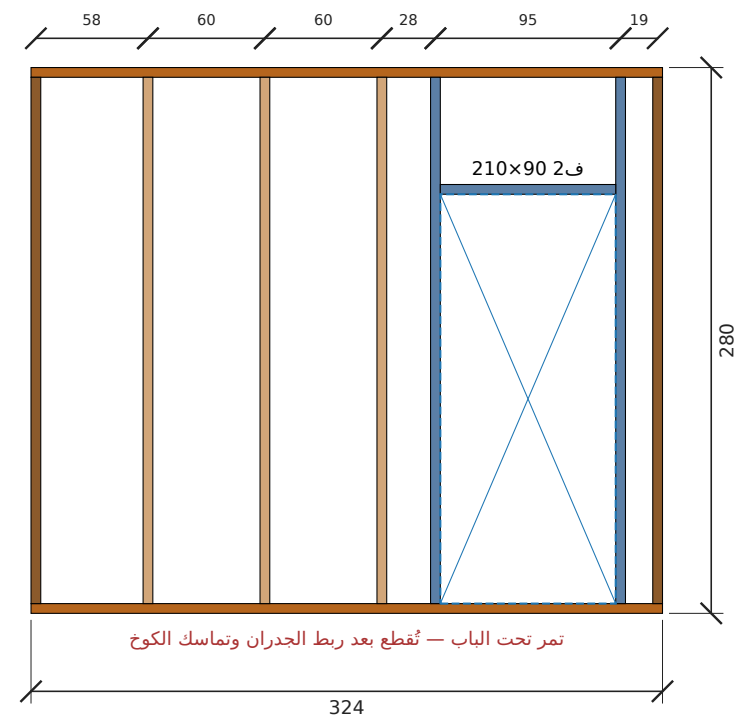
تأطير جدار ب-جناح الماستر — الطول 324 سم، الارتفاع 280 سم (داخلي)
