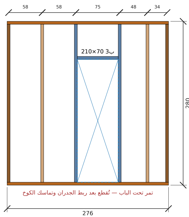
تأطير جدار ب-حمام الماستر — الطول 276 سم، الارتفاع 280 سم (داخلي)
