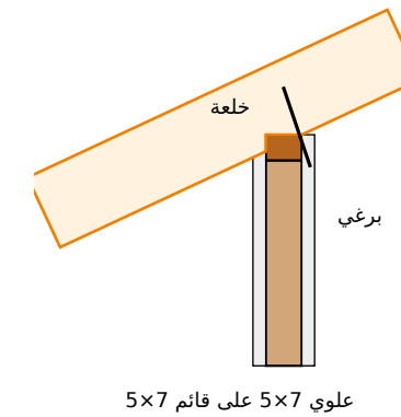
تفصيلة جلوس المداد على العلوي (1:5)
