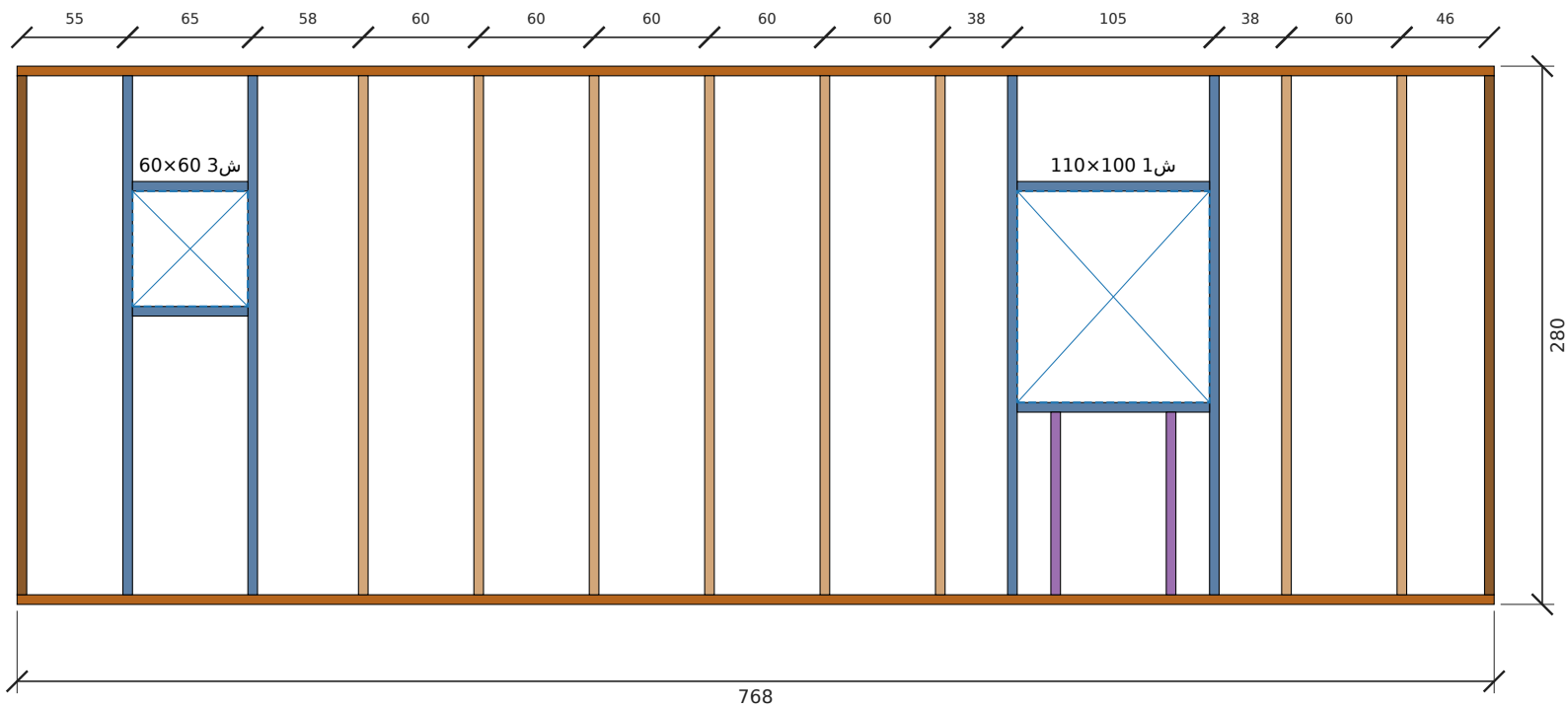
تأطير جدار ب-شرق — الطول 768 سم، الارتفاع 280 سم
