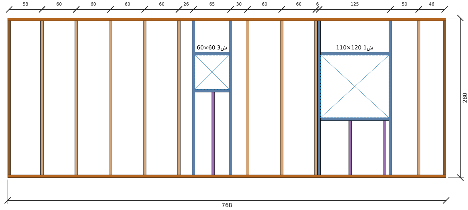
تأطير جدار أ-شمال — الطول 768 سم، الارتفاع 280 سم
