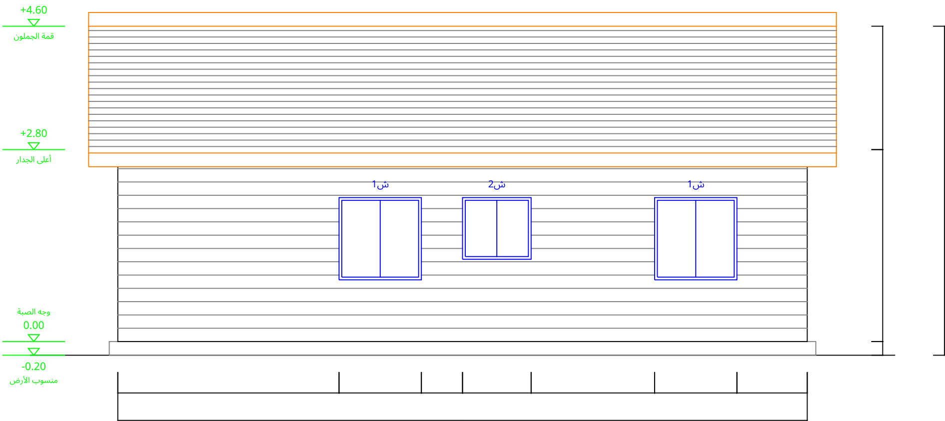
الواجهة الشرقية مقياس 1:50 | الوحدة: سم
