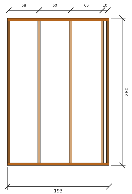
تأطير جدار د2-بين الحمامين — الطول 193 سم، الارتفاع 280 سم (داخلي)
