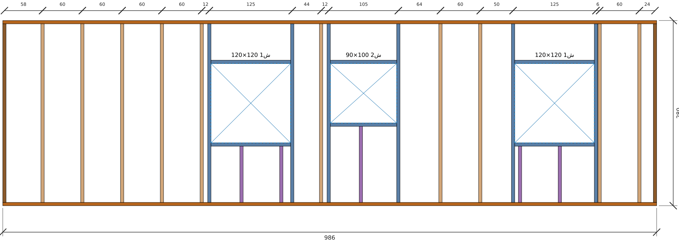
تأطير جدار شرق — الطول 986 سم، الارتفاع 280 سم
