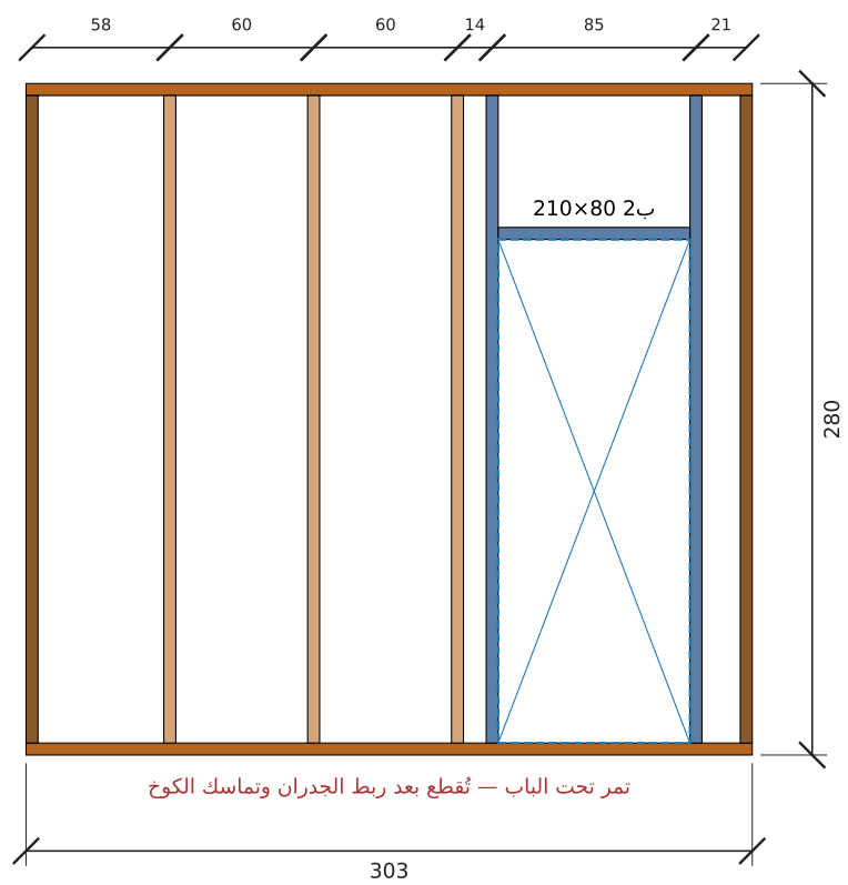
تأطير جدار د1-جنوب الحمامات — الطول 303 سم، الارتفاع 280 سم (داخلي)
