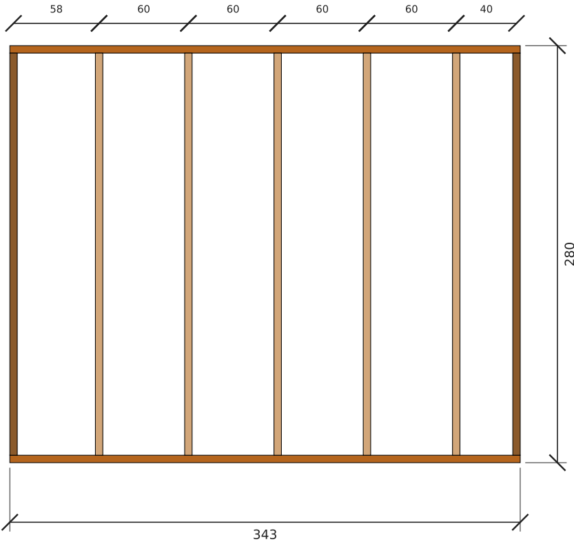
تأطير جدار د5-بين الغرفتين — الطول 343 سم، الارتفاع 280 سم (داخلي)
