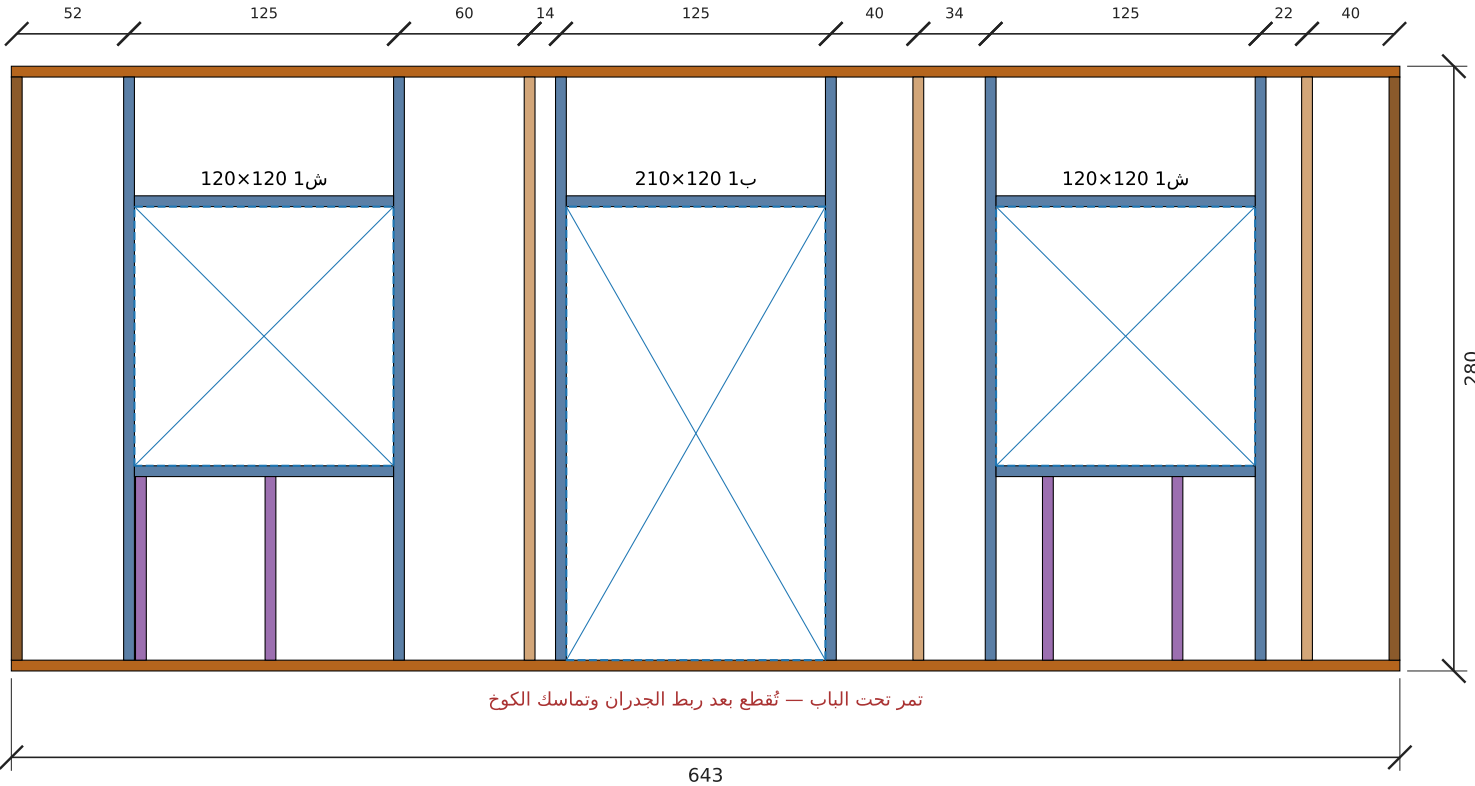
تأطير جدار جنوب — الطول 643 سم، الارتفاع 280 سم
