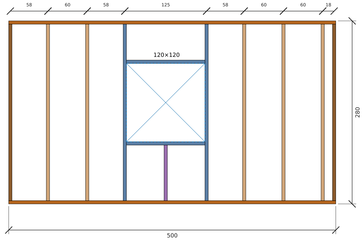
تأطير جدار W4-غرب — الطول 500 سم، الارتفاع 280 سم
