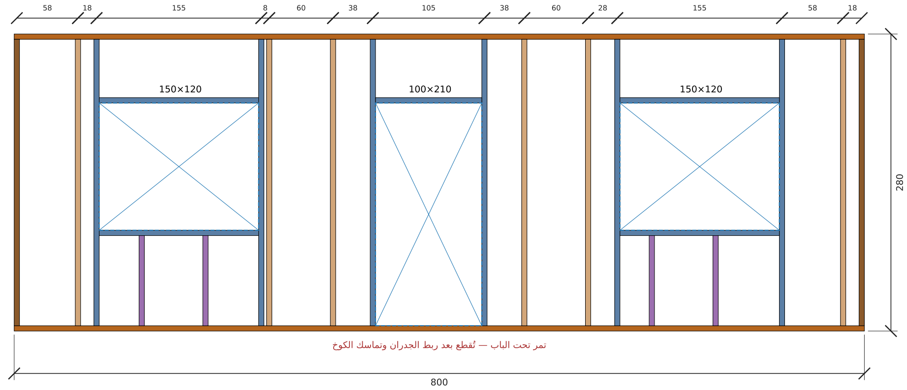
تأطير جدار W1-جنوب — الطول 800 سم، الارتفاع 280 سم
