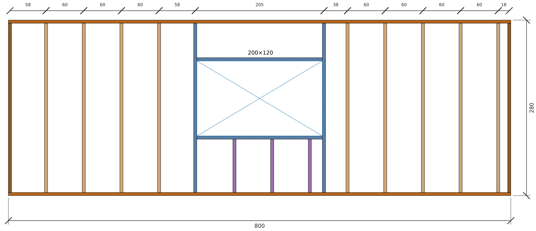
تأطير جدار W3-شمال — الطول 800 سم، الارتفاع 280 سم
