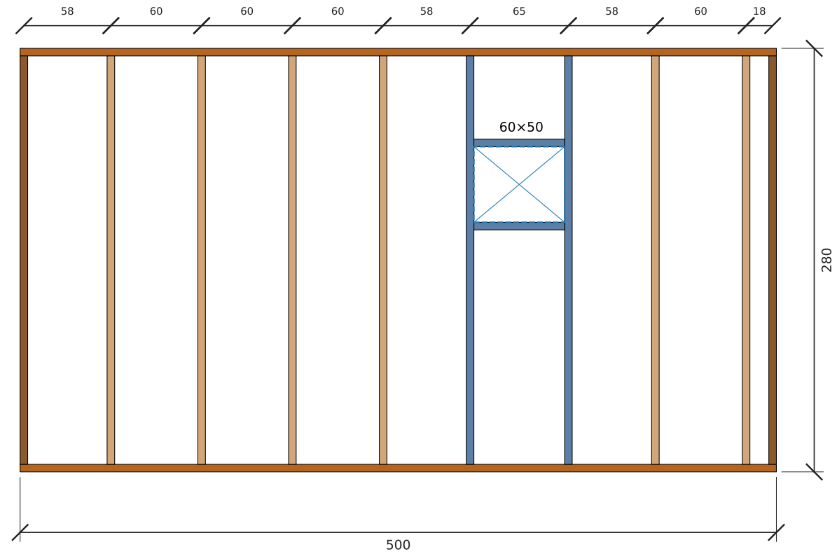
تأطير جدار W2-شرق — الطول 500 سم، الارتفاع 280 سم
