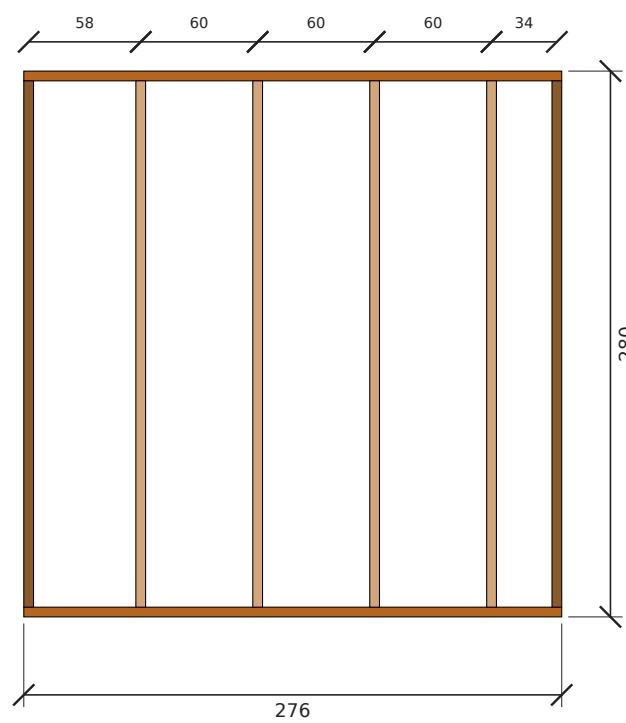
تأطير جدار د2-جدار الحمام — الطول 276 سم، الارتفاع 280 سم (داخلي)
