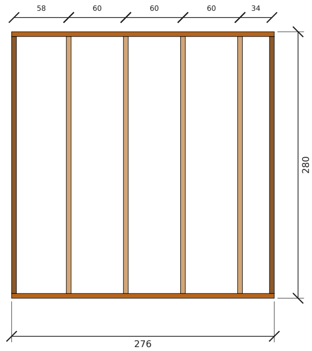
تأطير جدار د2-جدار الحمام — الطول 276 سم، الارتفاع 280 سم (داخلي)
