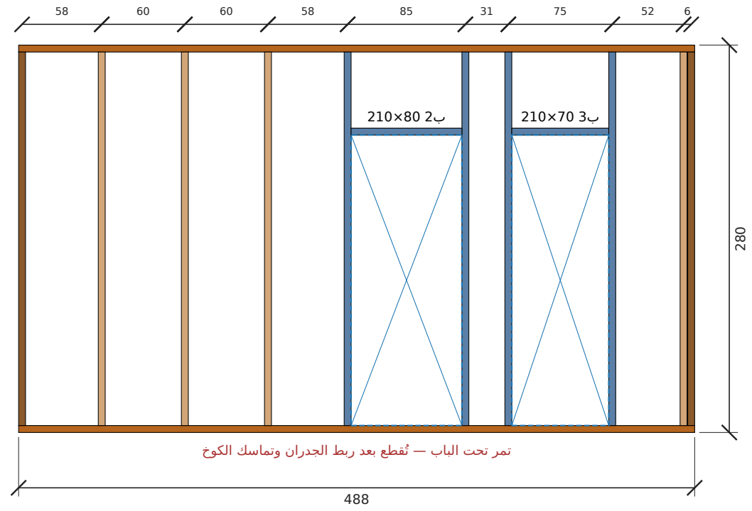
تأطير جدار د1-فاصل الصالة — الطول 488 سم، الارتفاع 280 سم (داخلي)
