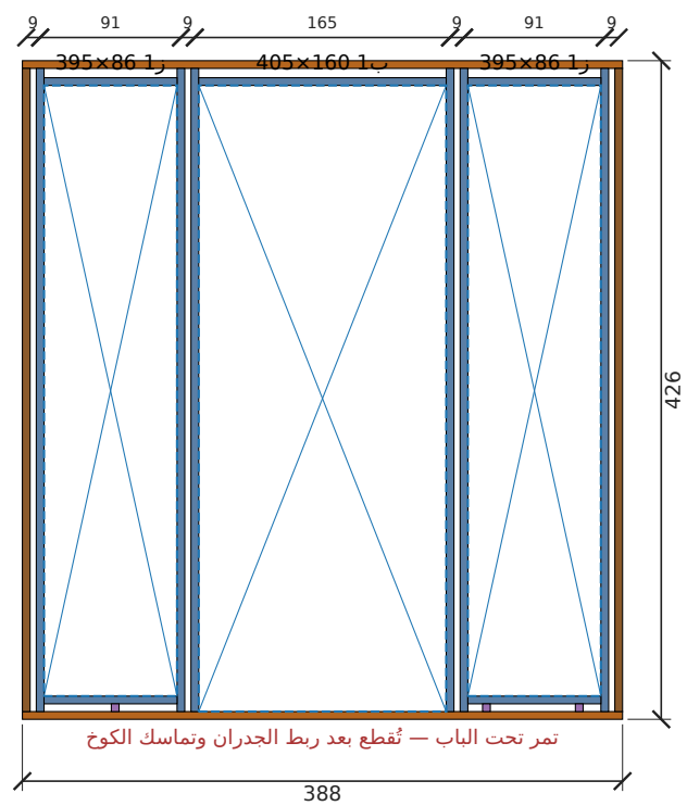
تأطير جدار جنوب — الطول 388 سم، الارتفاع 426 سم
