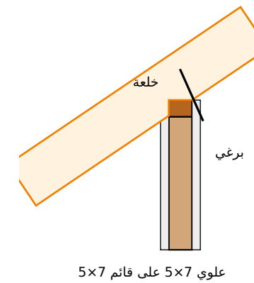
تفصيلة جلوس المداد على العلوي (1:5)
